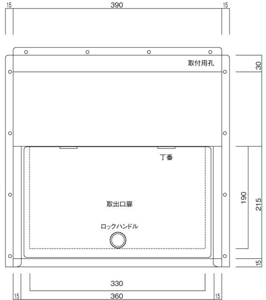
裏面図
