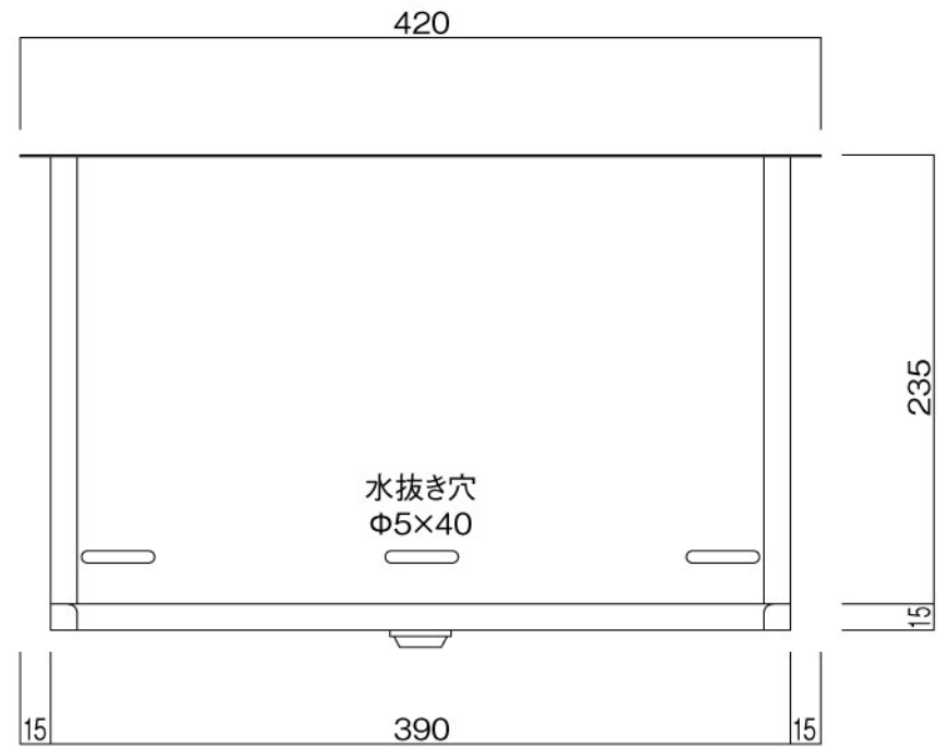
底面図
