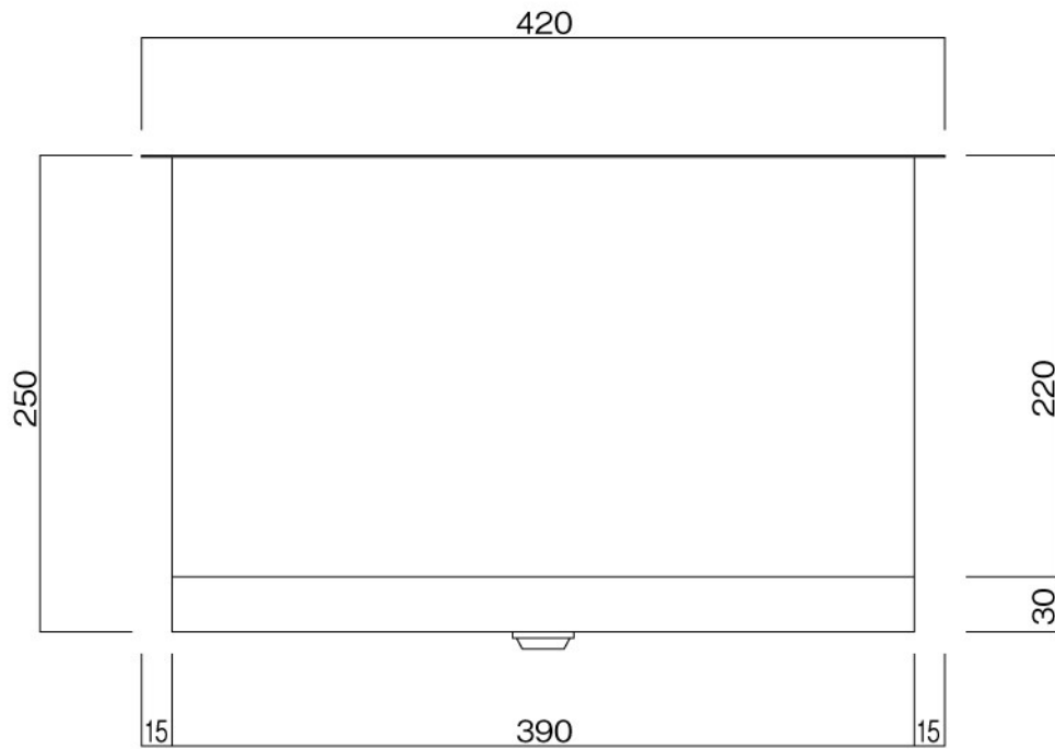
平面図
