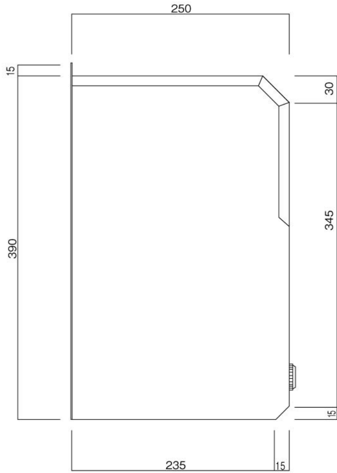
側面図
