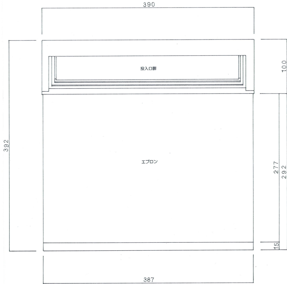
正面図
