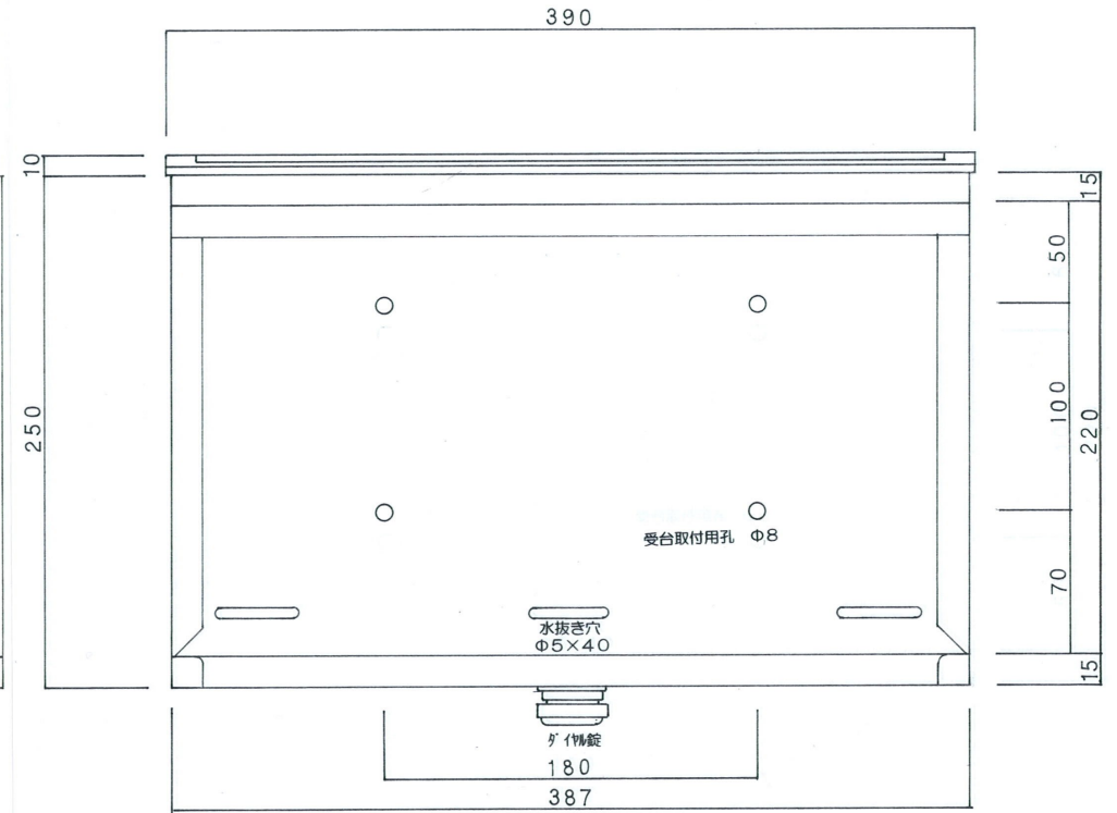
底面図
