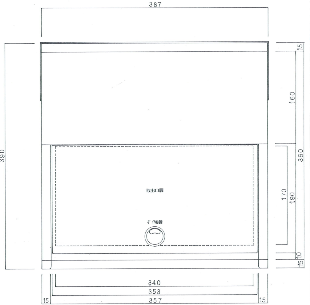
裏面図
