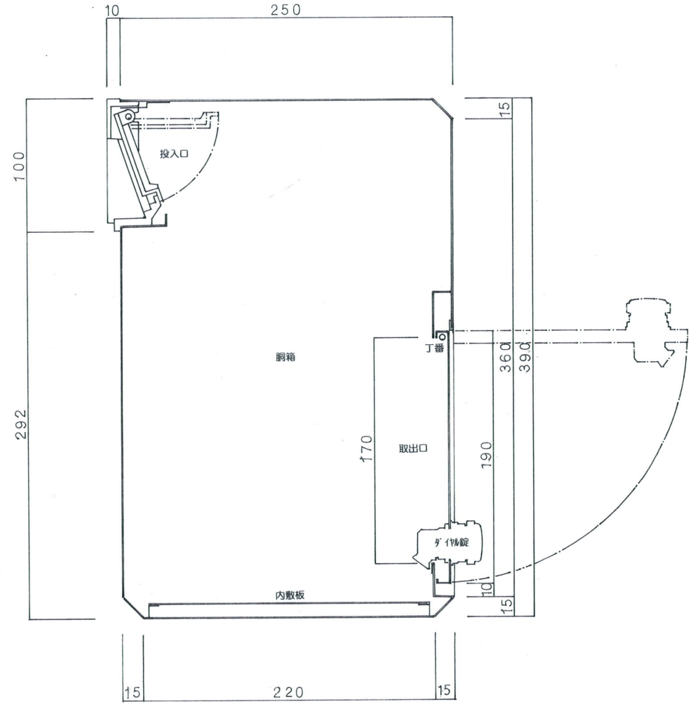
縦断面図
