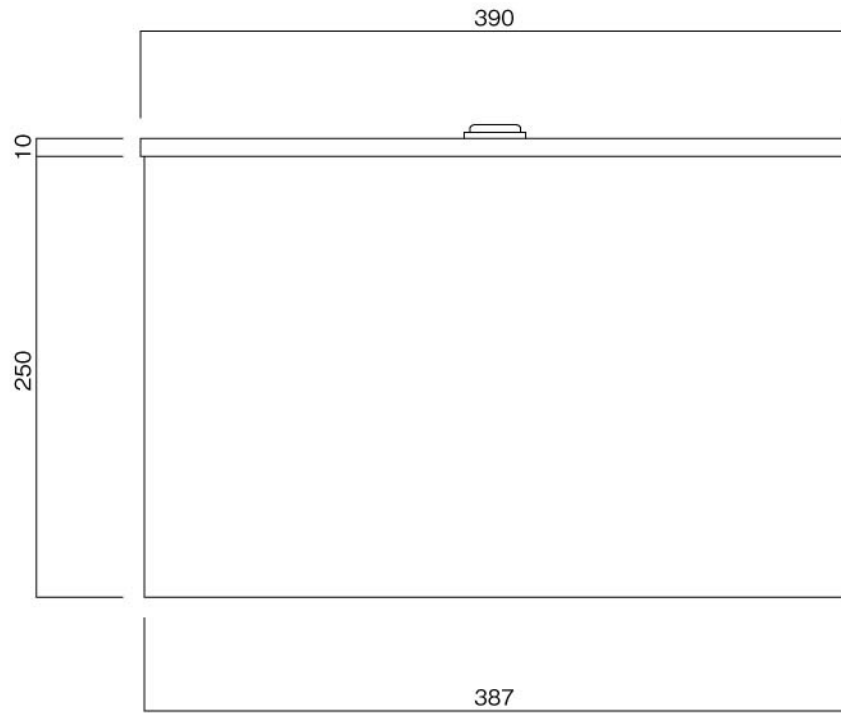
平面図
