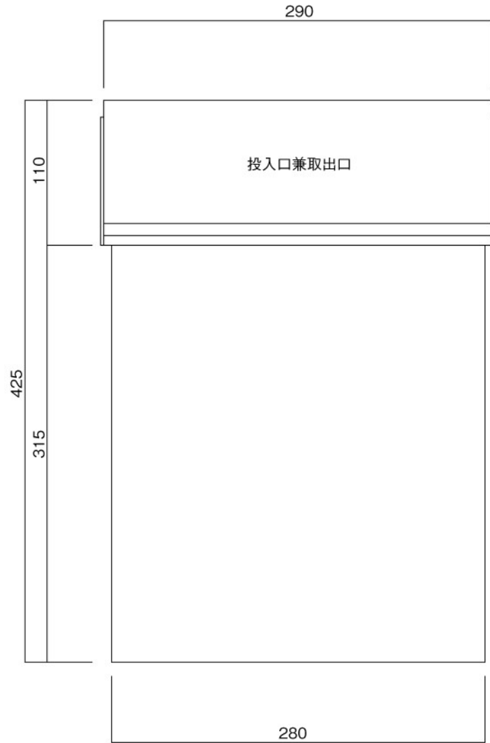
正面図
