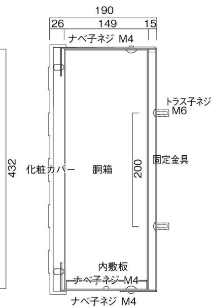
縦断面図
