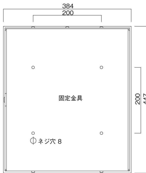
裏面図
