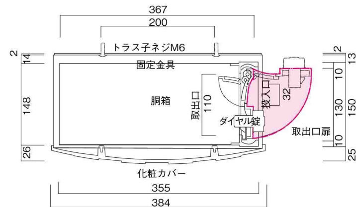
横断面図
