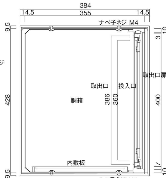
縦断面図
