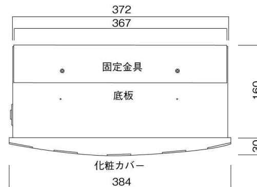
底面図
