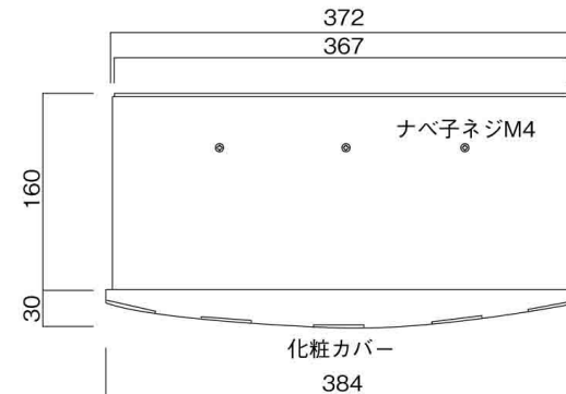
平面図
