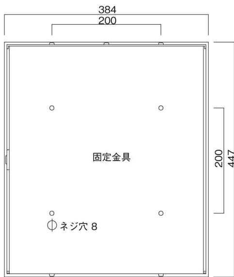
裏面図
