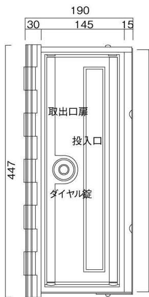
左側面図
