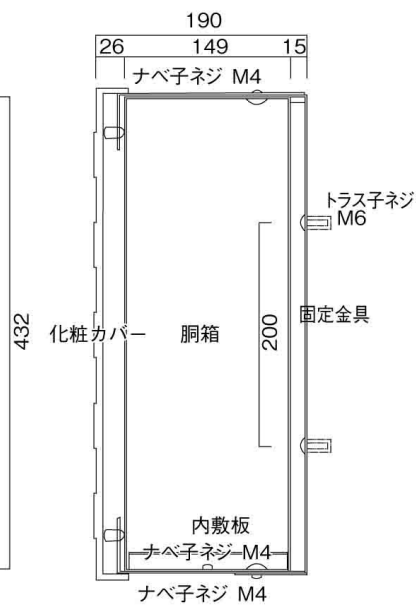
縦断面図
