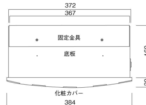
化粧カバー
