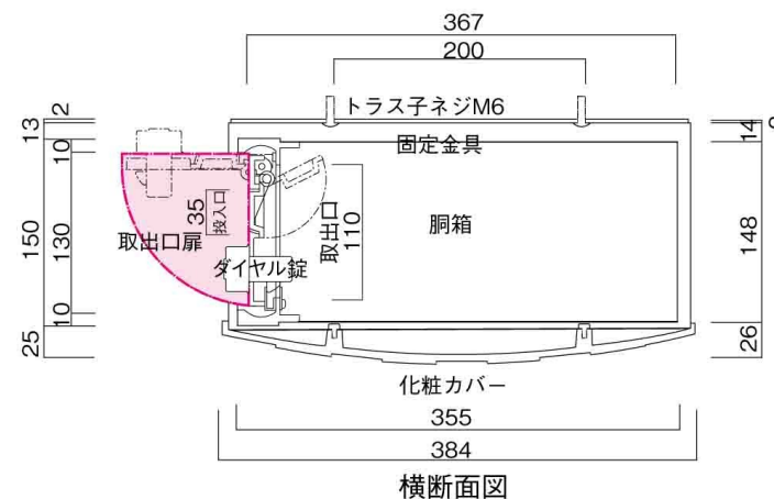
化粧カバー
