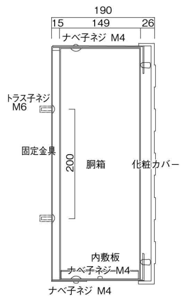
縦断面図
