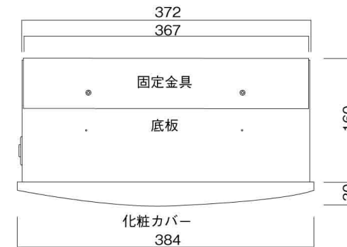
底面図
