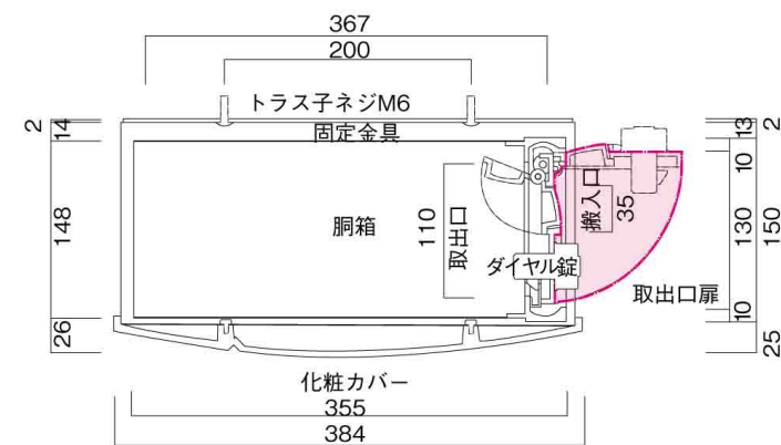
横断面図
