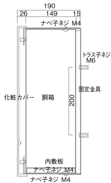
縦断面図
