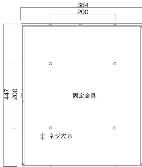
裏面図
