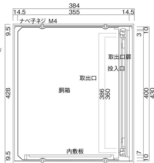
縦断面図
