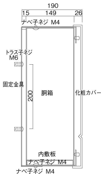
縦断面図
