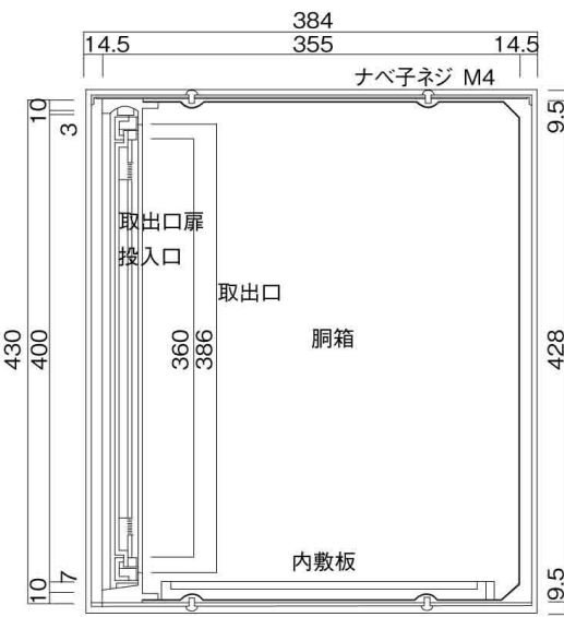
縦断面図
