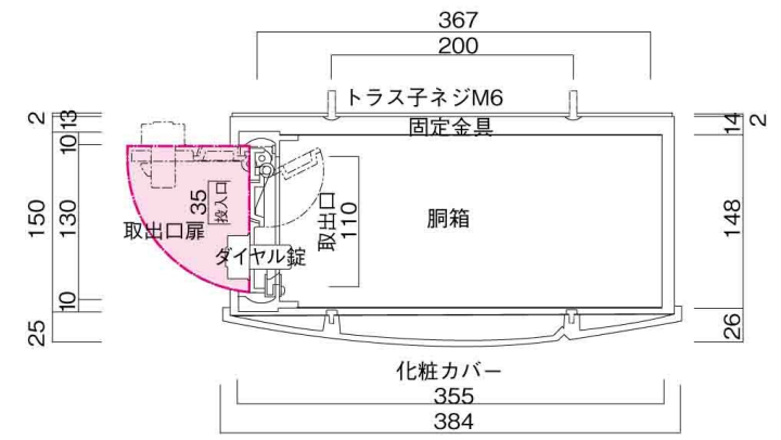
横断面図
