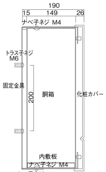
縦断面図
