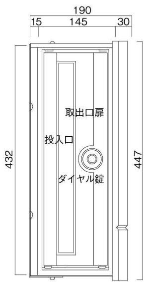
左側面図
