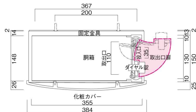
横断面図
