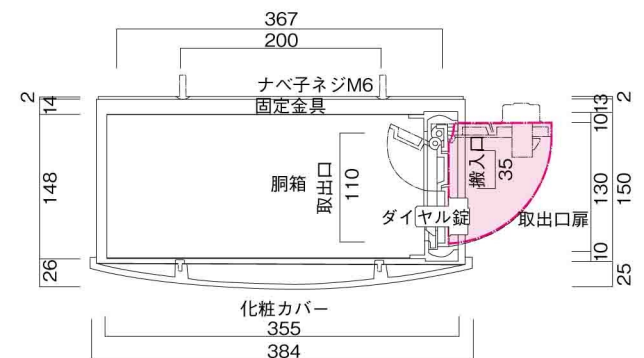
横断面図
