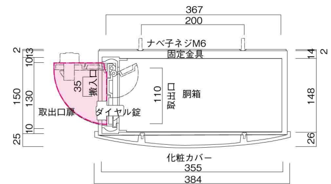
横断面図
