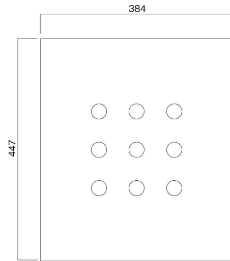
正面図
