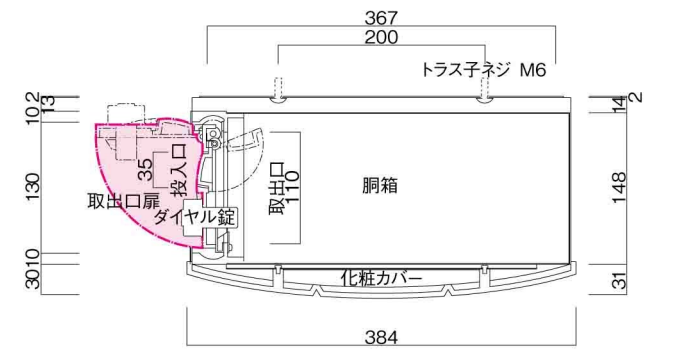
横断面図
