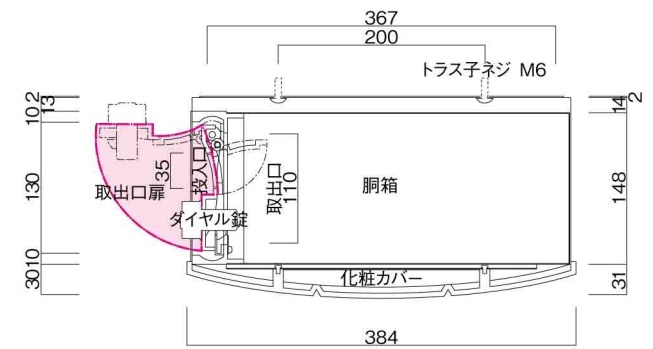
横断面図
