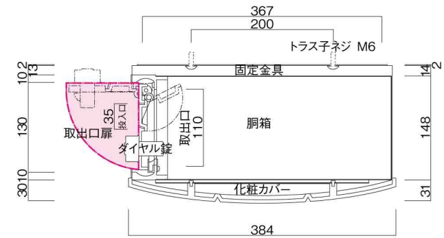
横断面図
