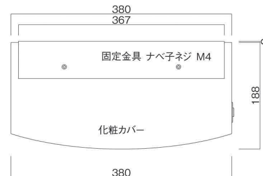
底面図
