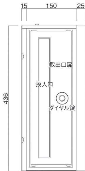
左側面図
