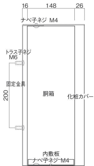
縦断面図
