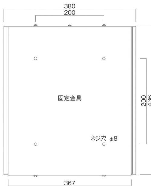
裏面図
