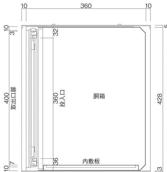
縦断面図
