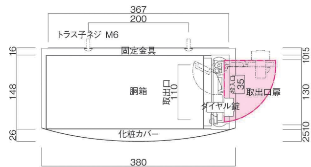
横断面図
