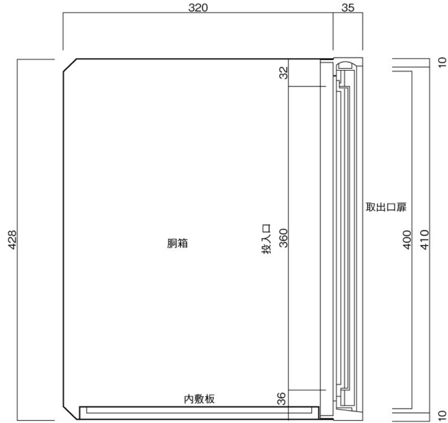
縦断面図
