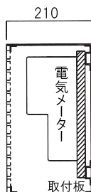
縦断面図
