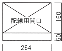
底面図
