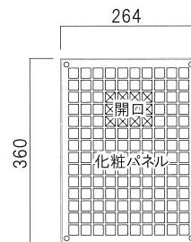
正面図
