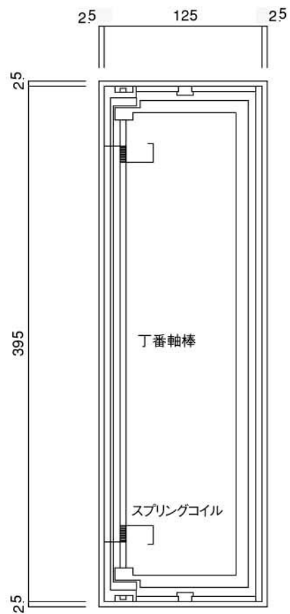
裏面図
