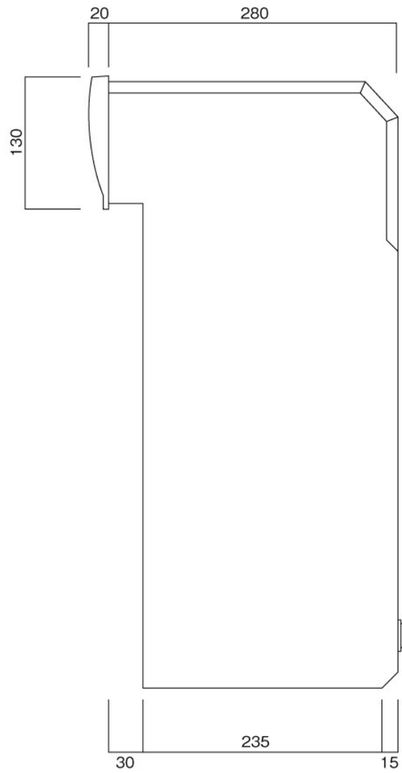
側面図
