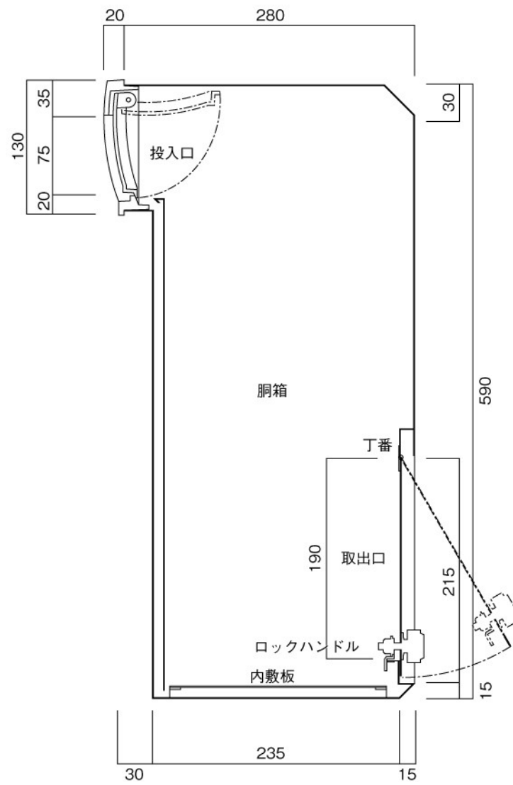
縦断面図
