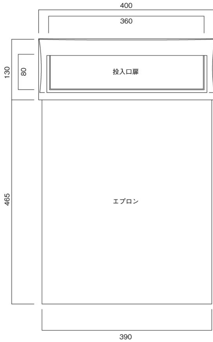
正面図
