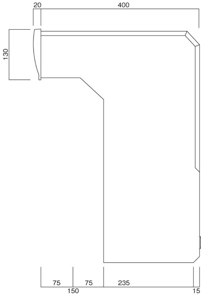
側面図
