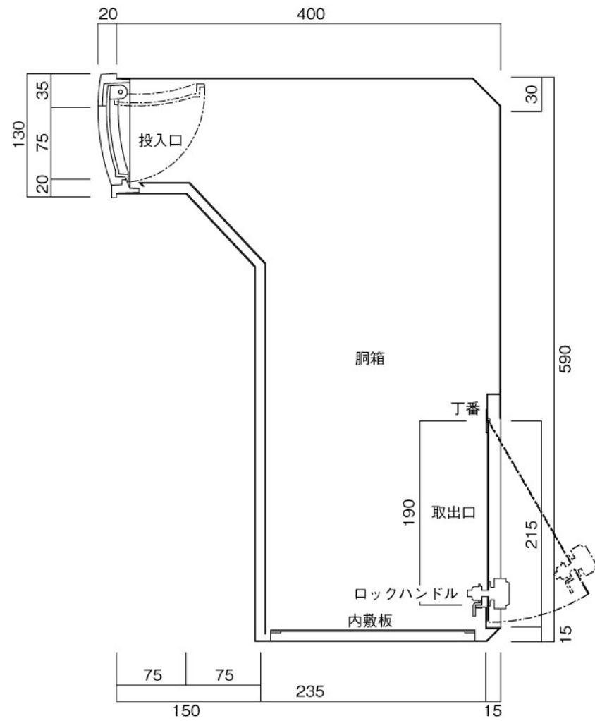
縦断面図
