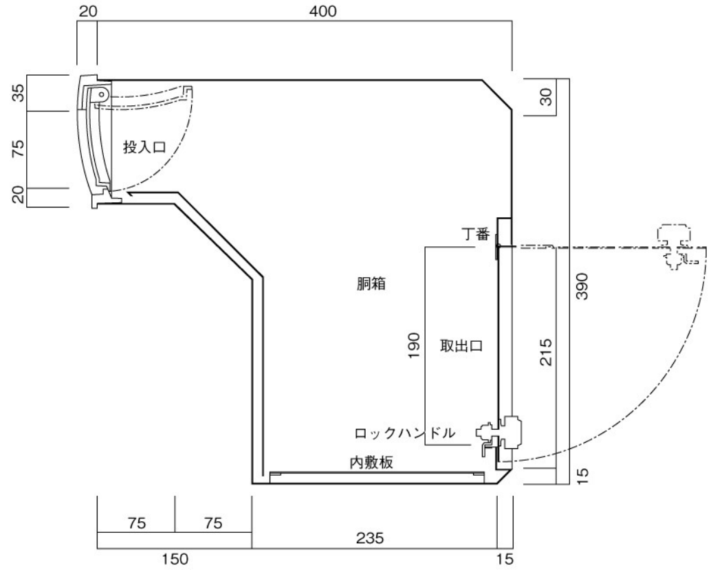
縦断面図
