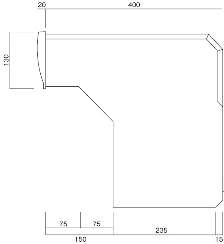
側面図
