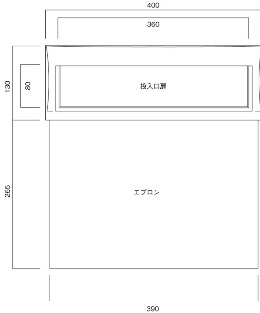
正面図
