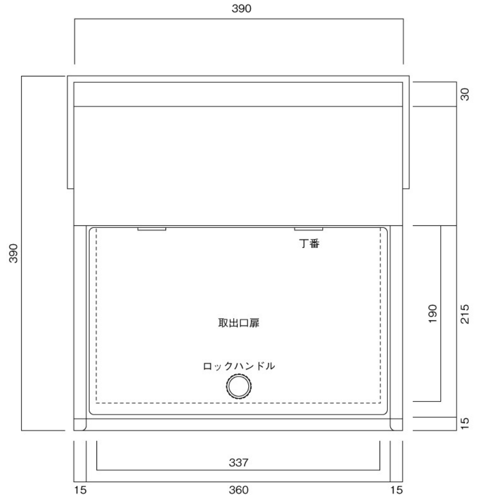
裏面図
