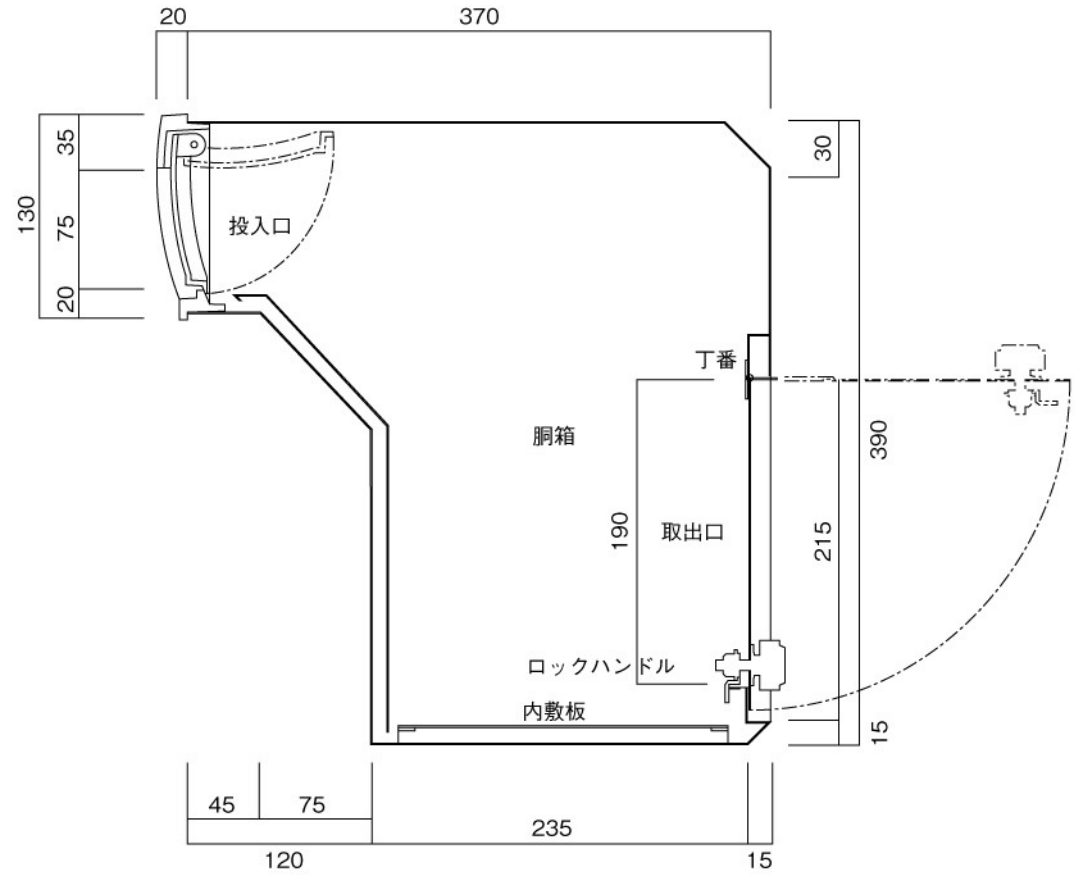
縦断面図
