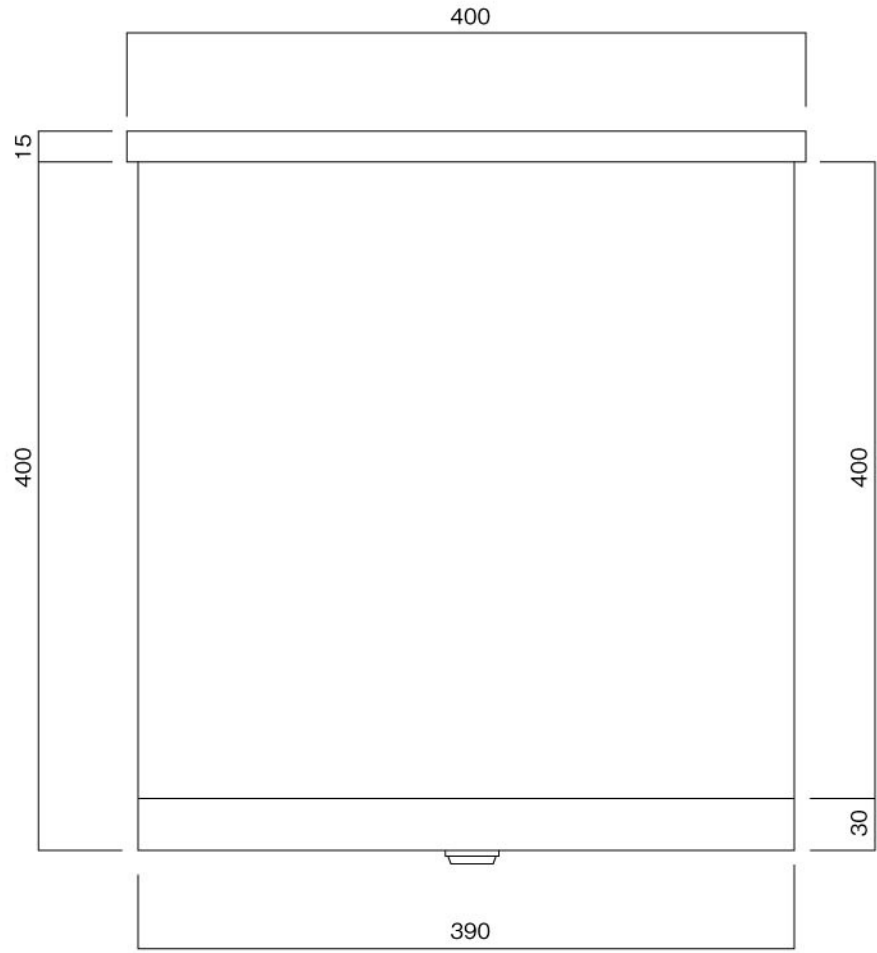
平面図
