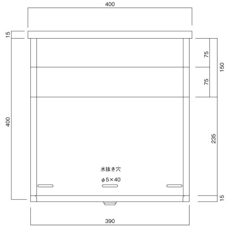
底面図
