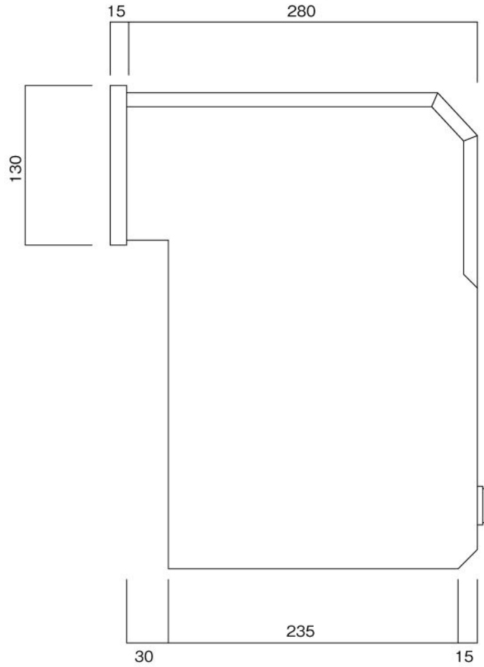
側面図
