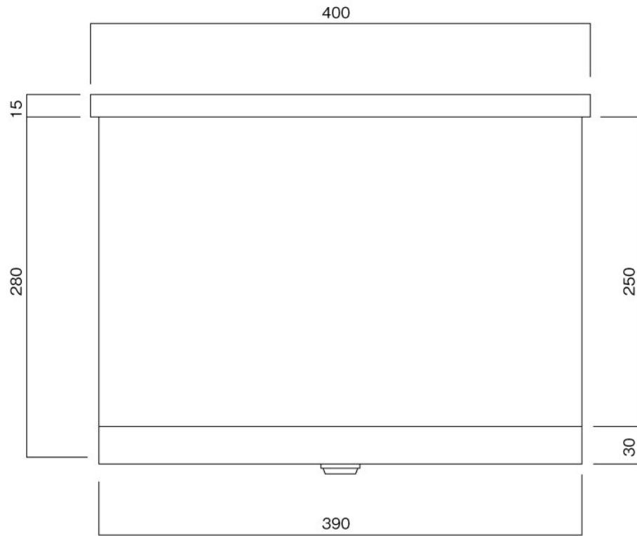
平面図
