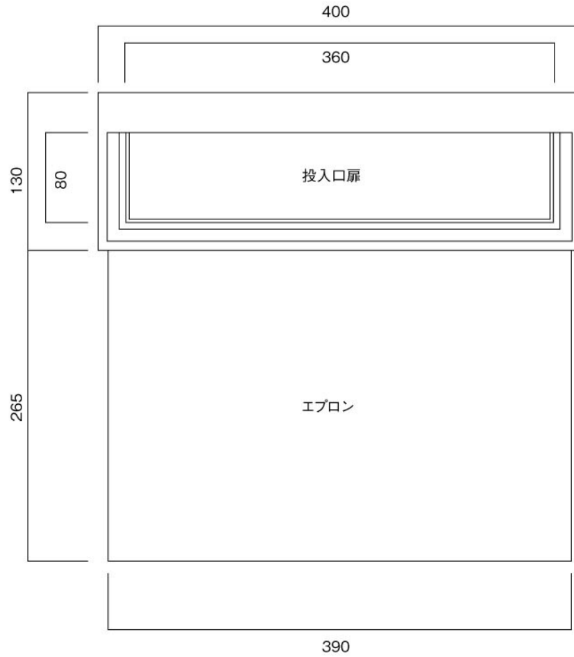
正面図
