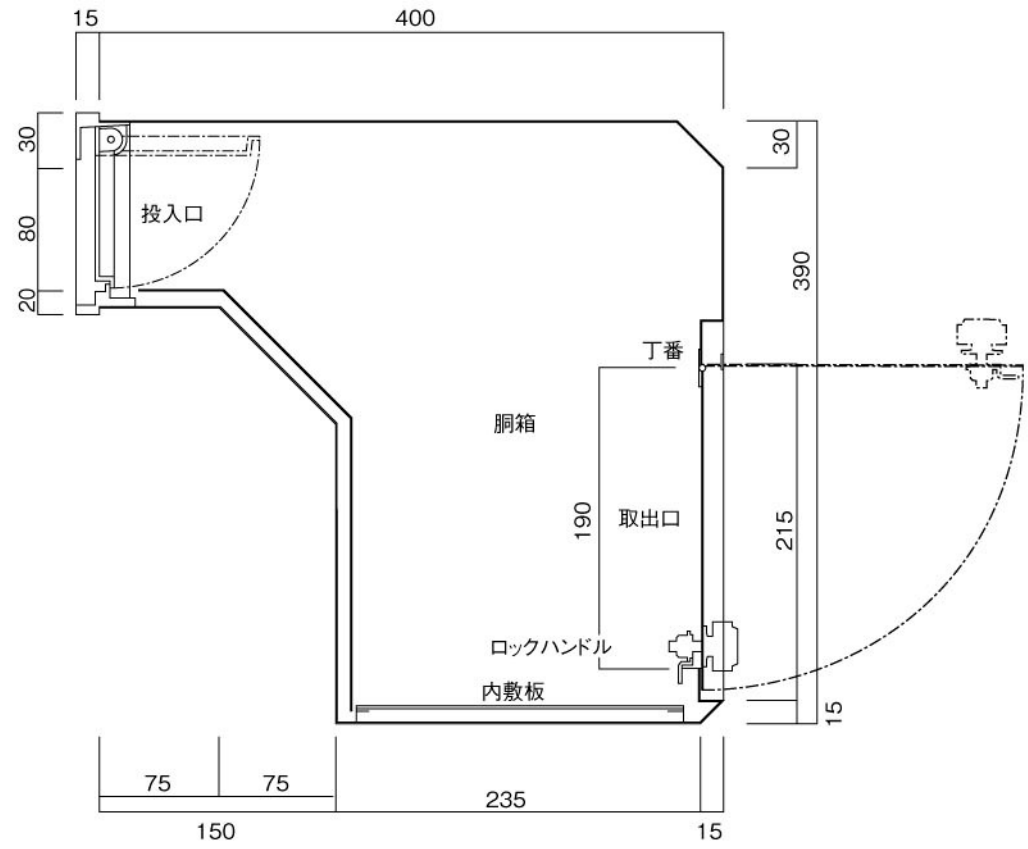
縦断面図
