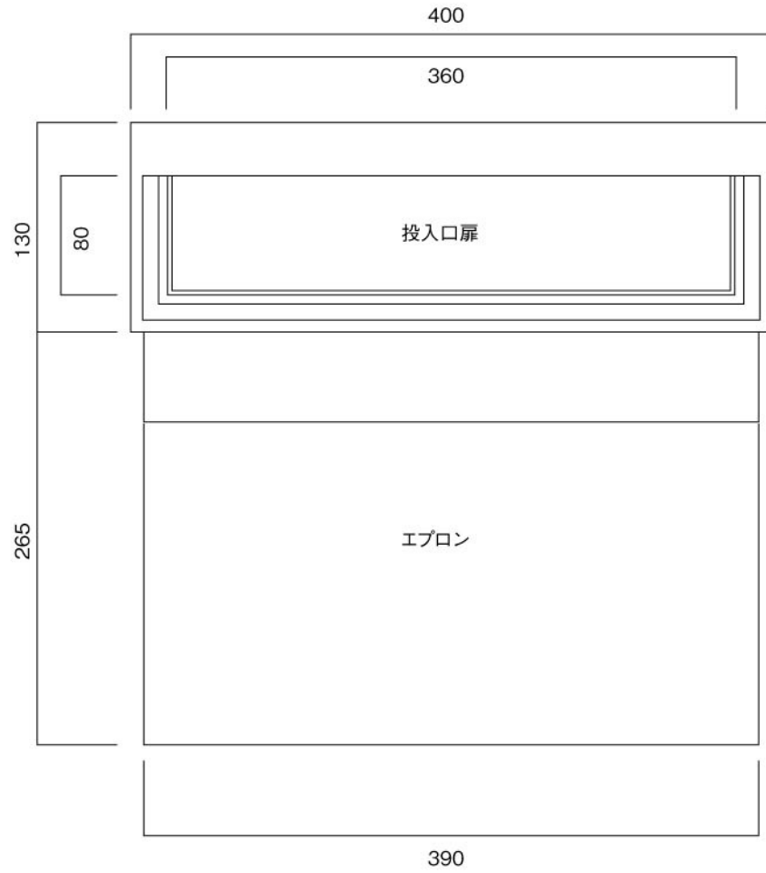
正面図
