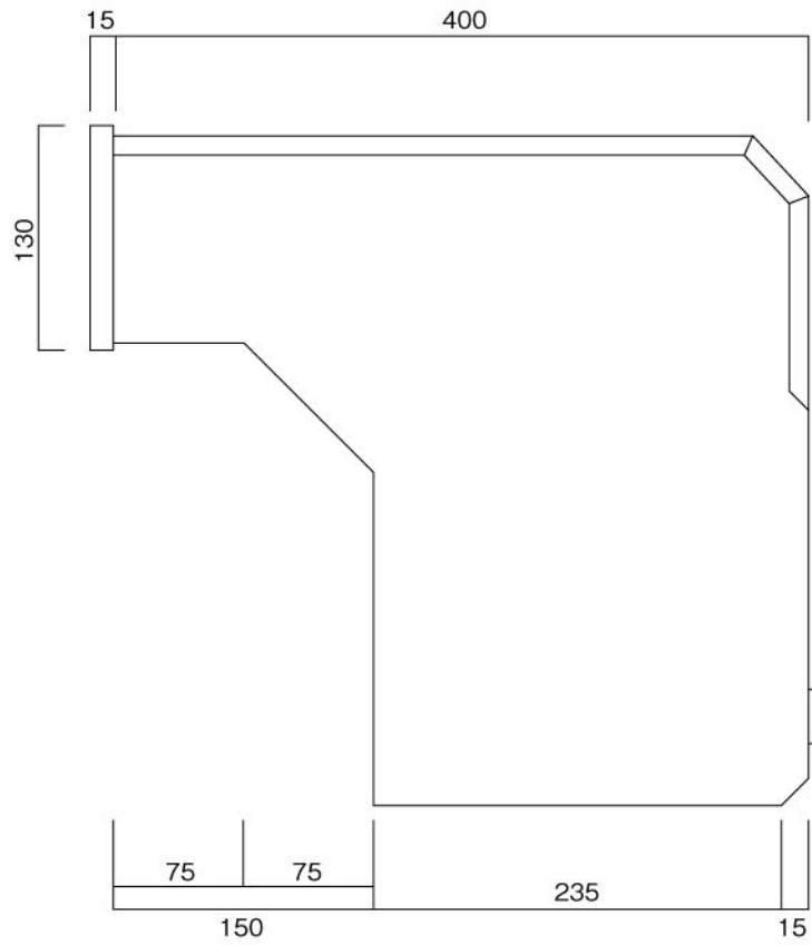
側面図
