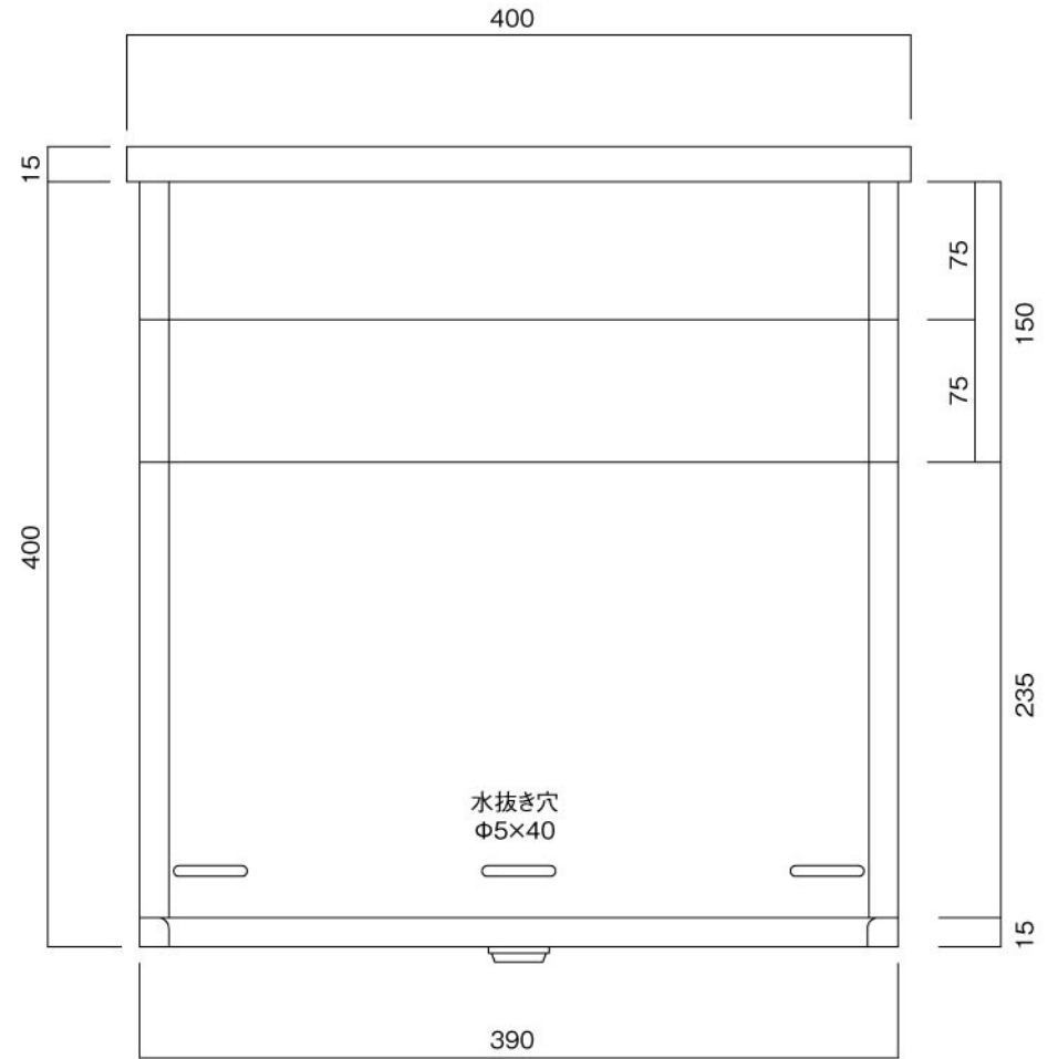
底面図
