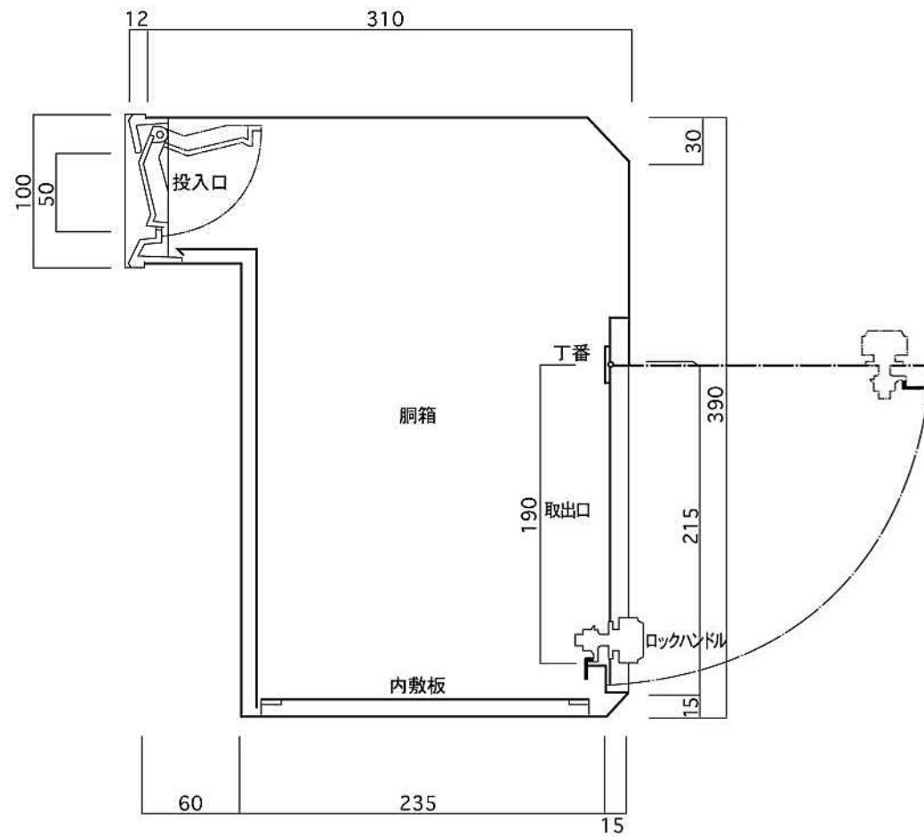
縦断面図
