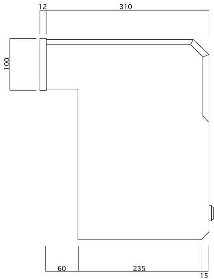
側面図
