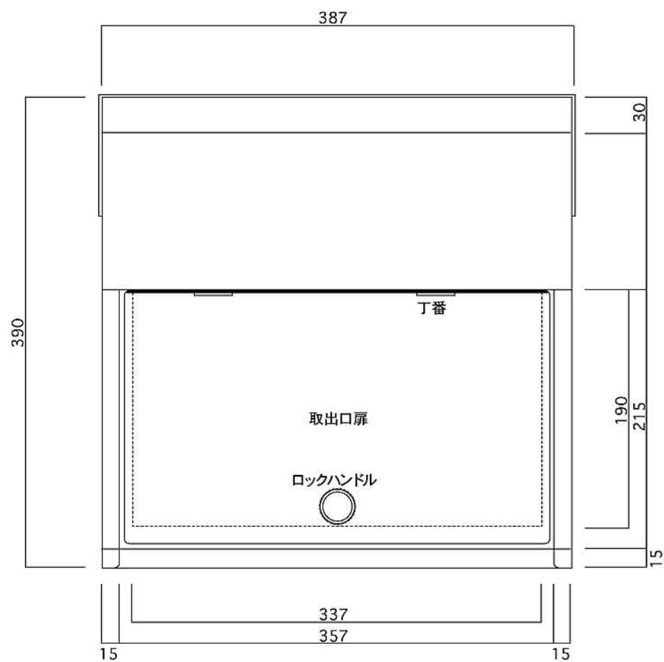
裏面図
