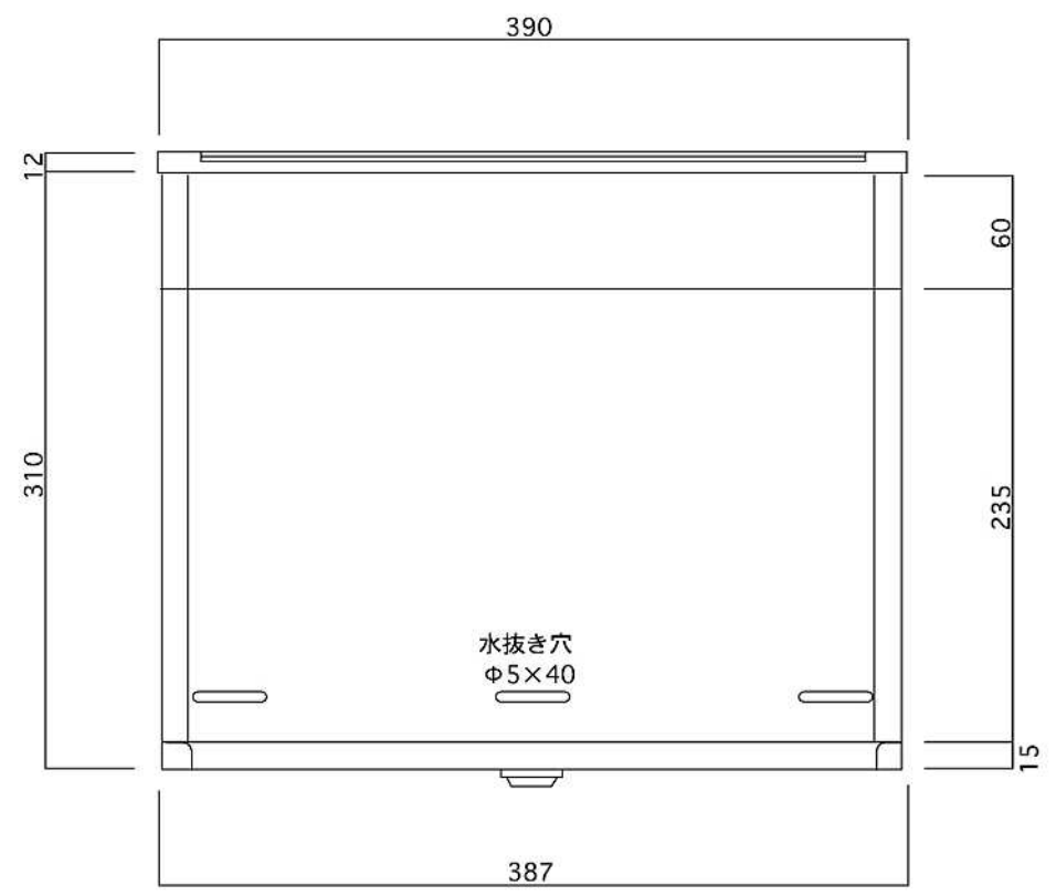
底面図
