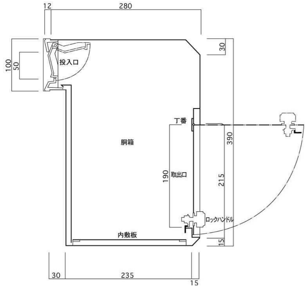
縦断面図
