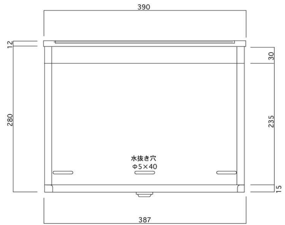
底面図
