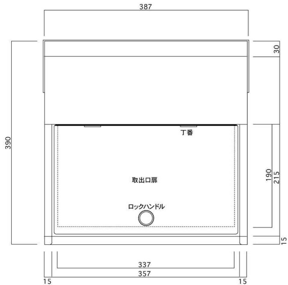
裏面図
