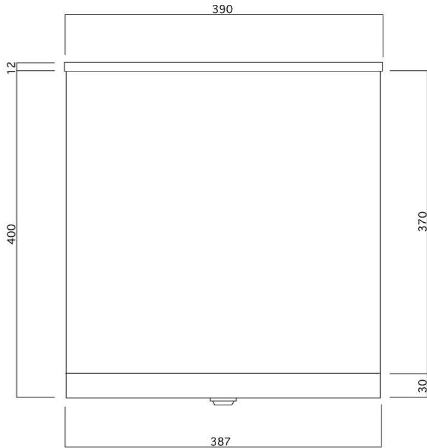
平面図
