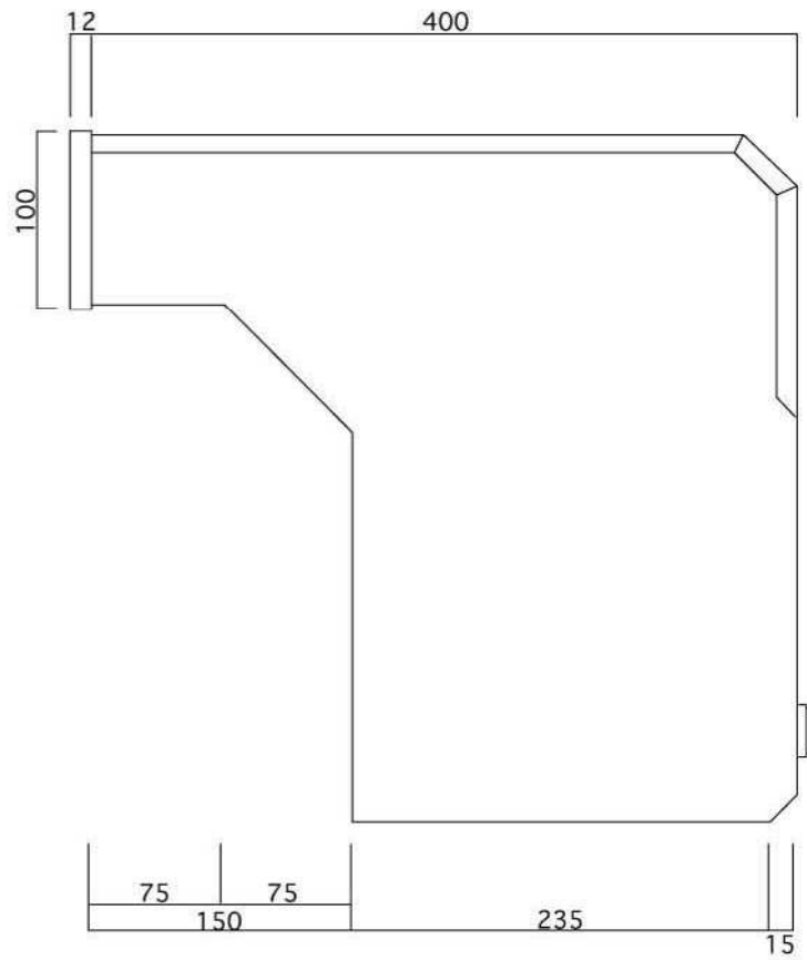
側面図
