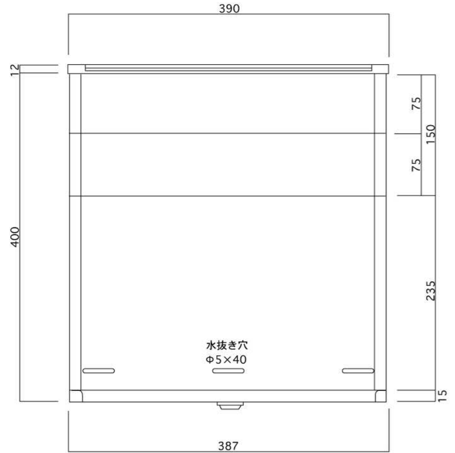
底面図
