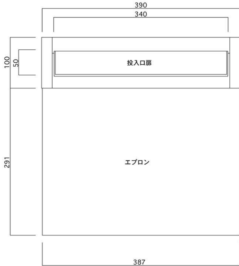
正面図
