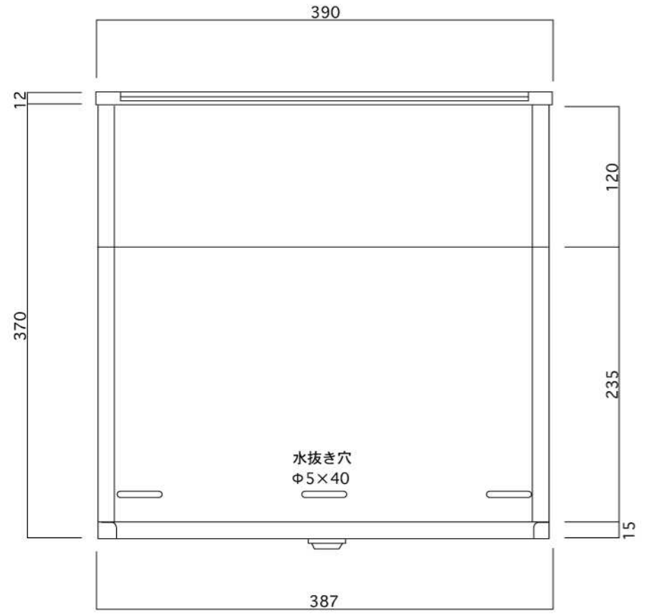
底面図
