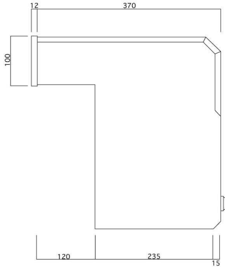
側面図
