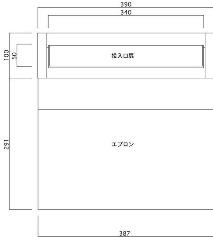
正面図
