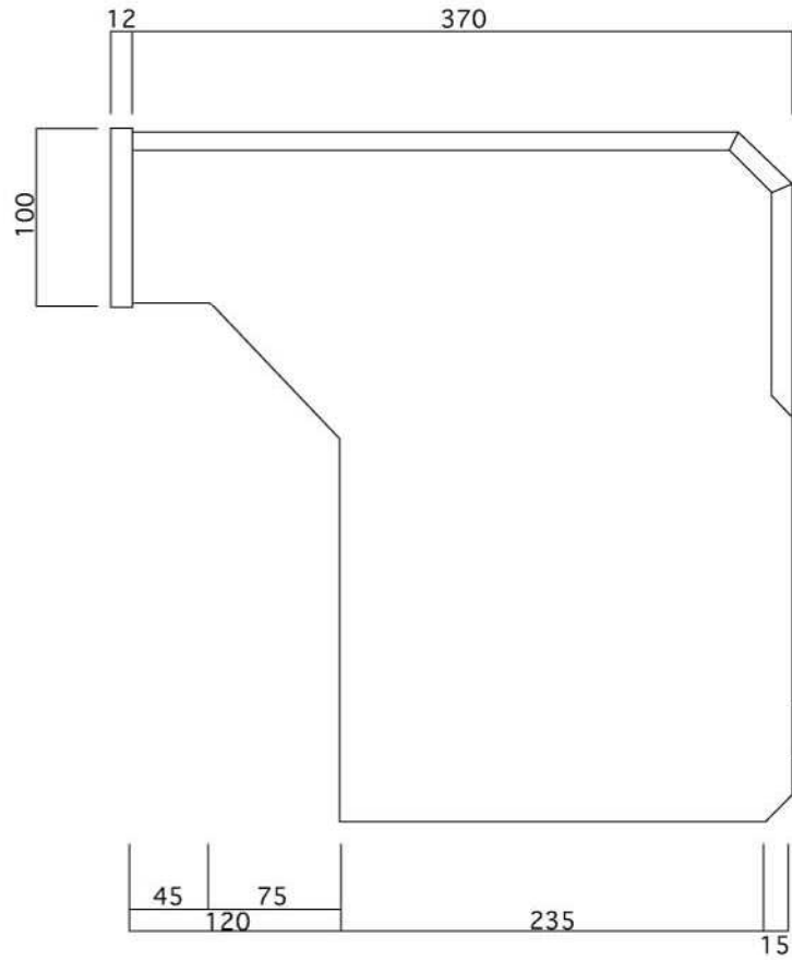
側面図
