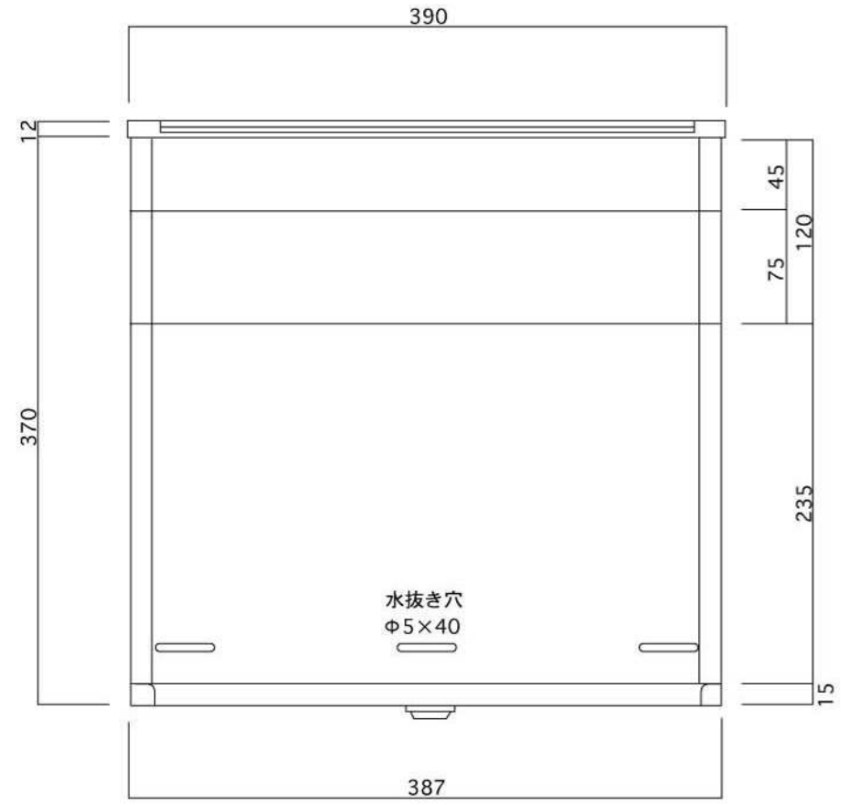
底面図
