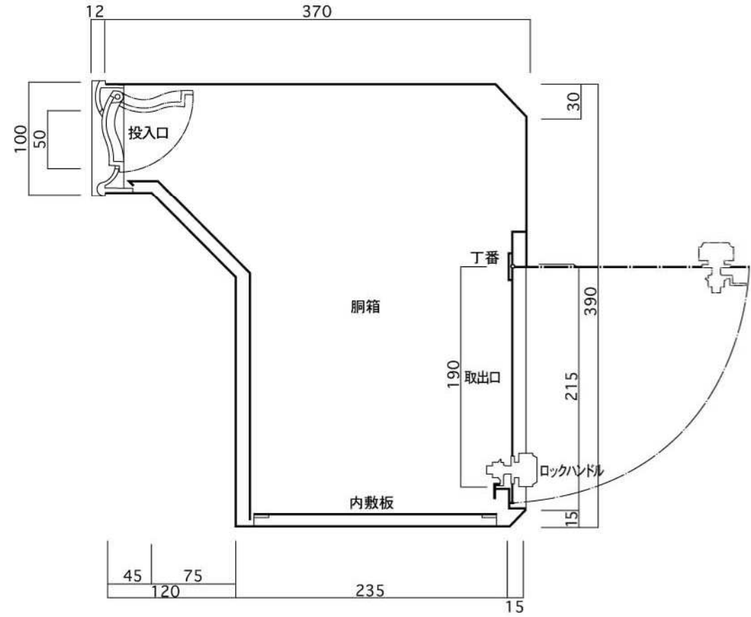
縦断面図
