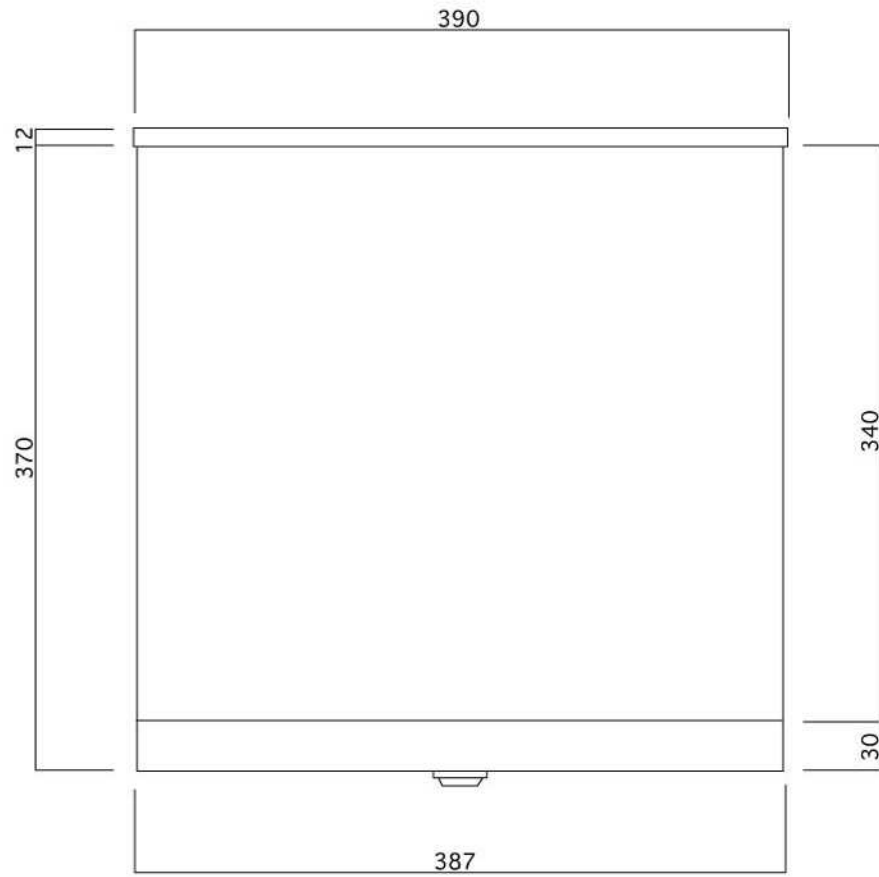
平面図
