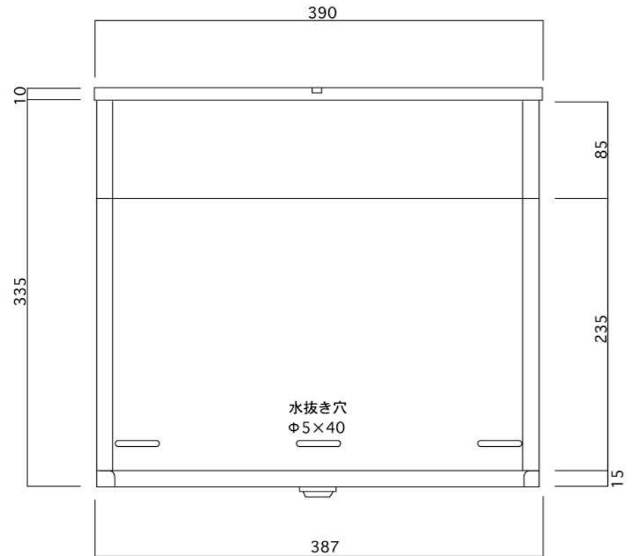
底面図
