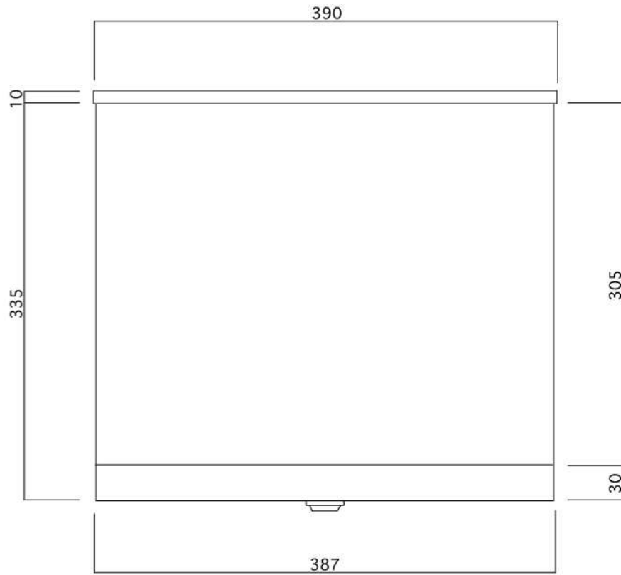
平面図
