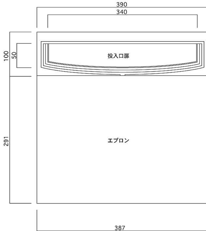
正面図
