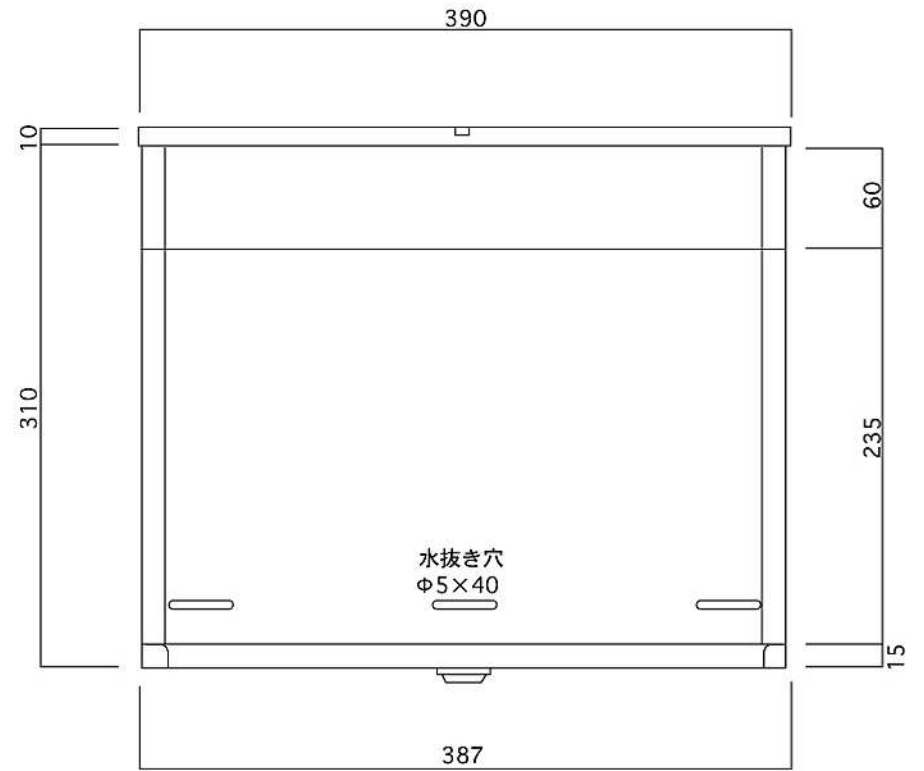
底面図
