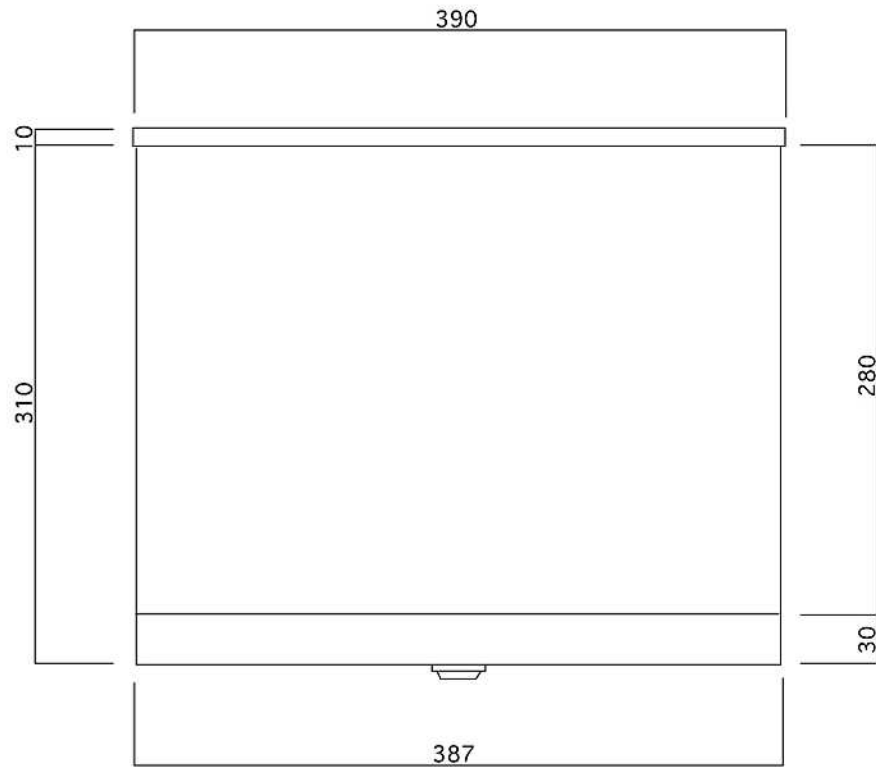
平面図
