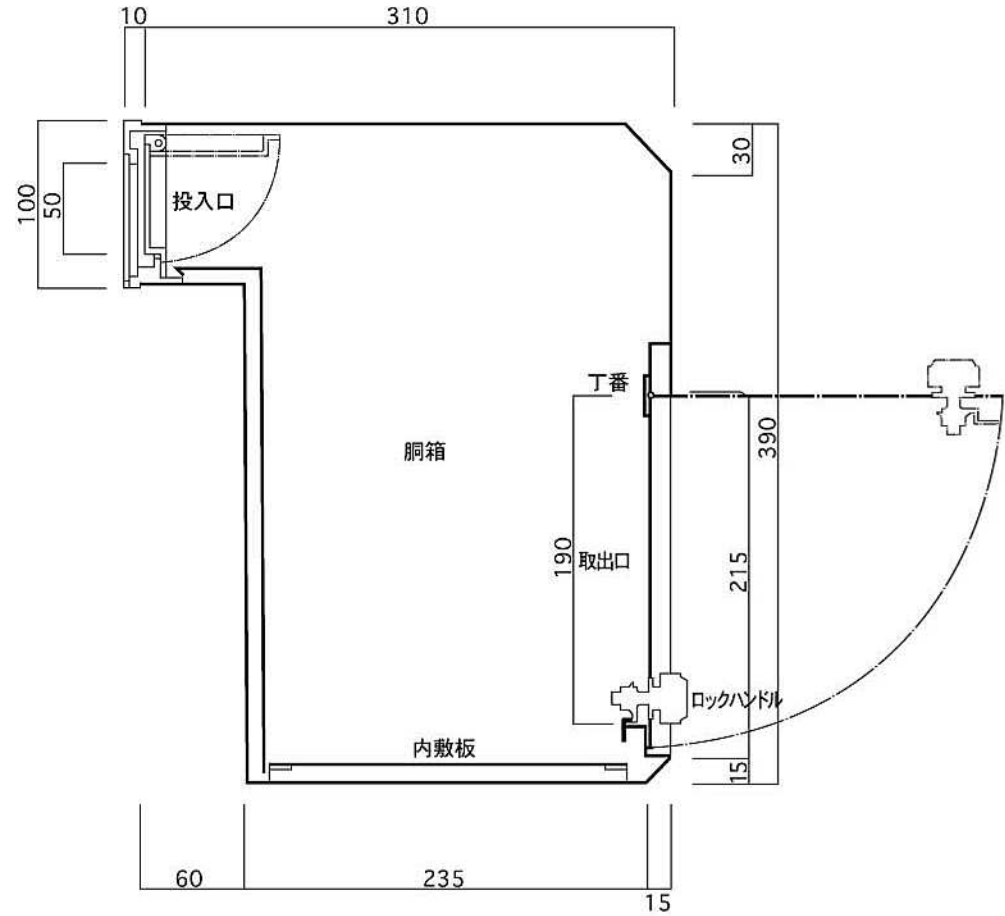
縦断面図
