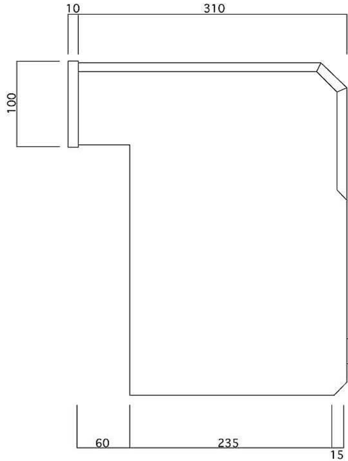
側面図
