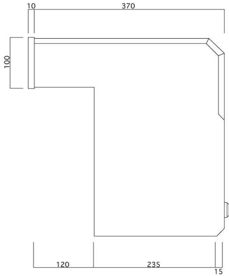
側面図
