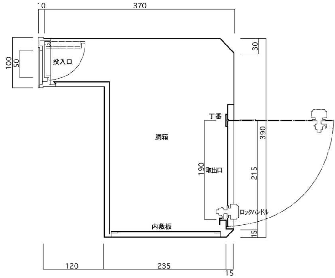
縦断面図
