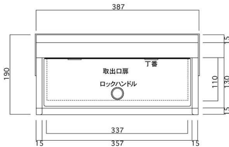
裏面図
