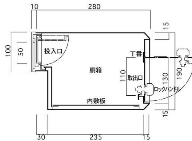
縦断面図
