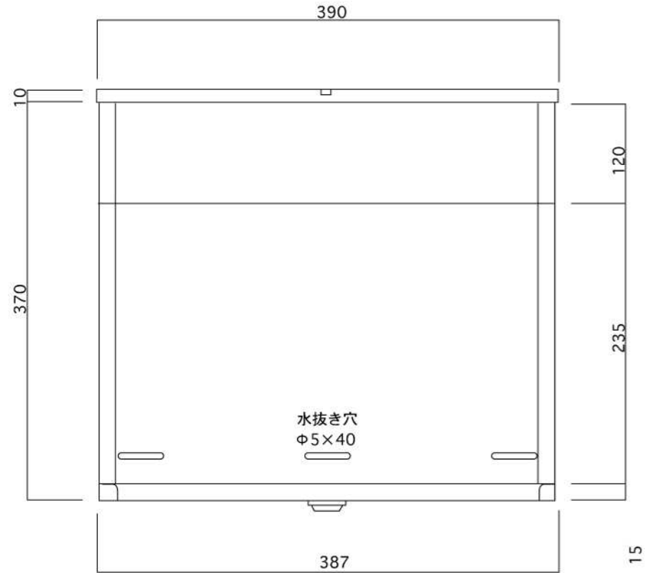
底面図
