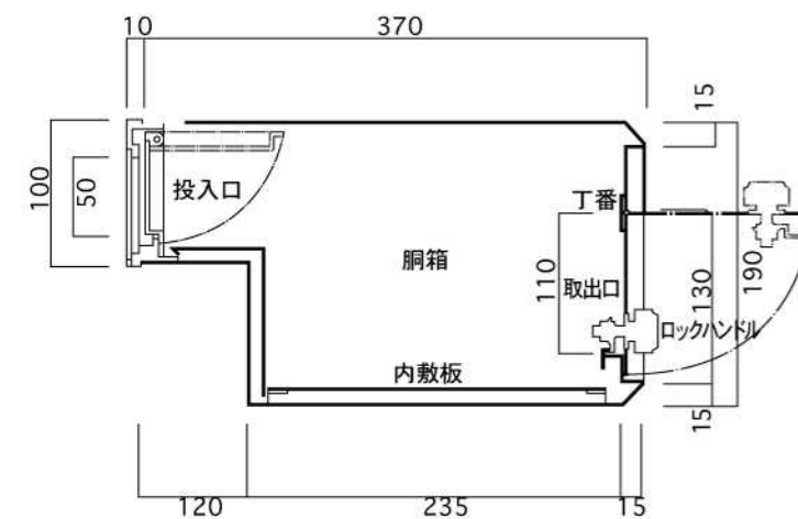
縦断面図
