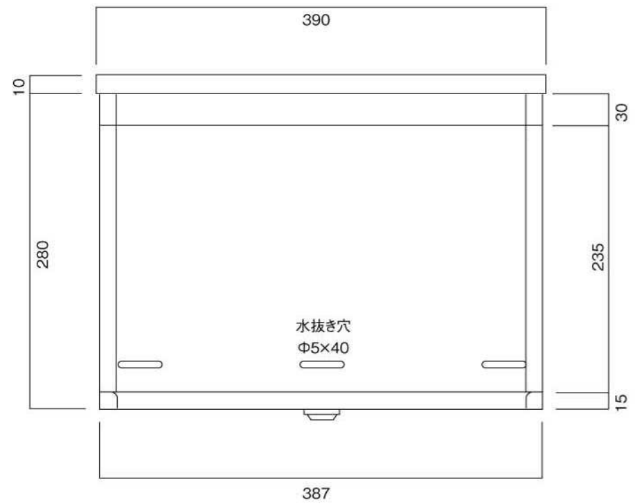
底面図
