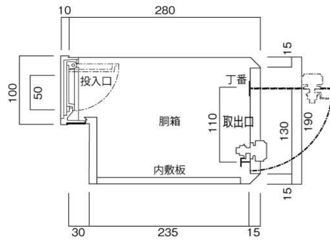
縦断面図
