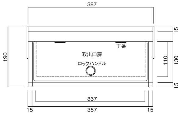
裏面図
