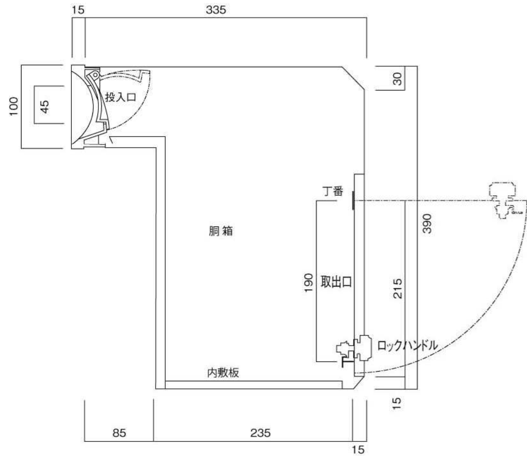
縦断面図
