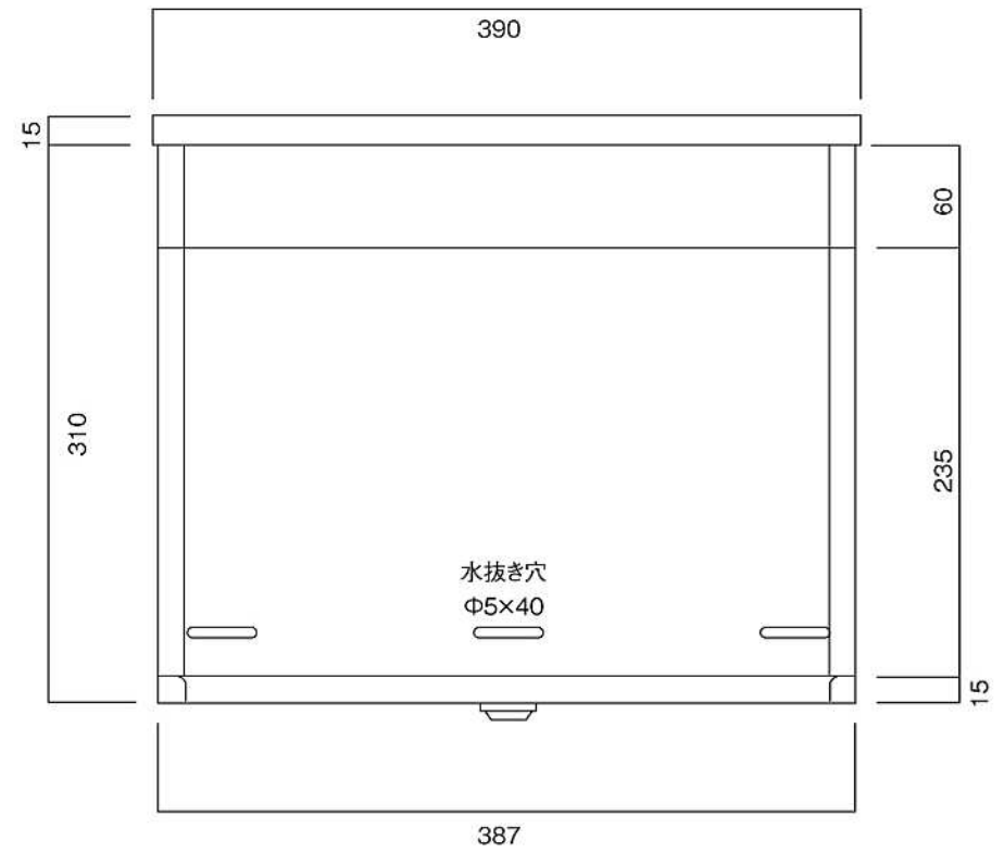
底面図
