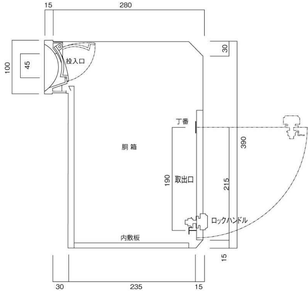
縦断面図
