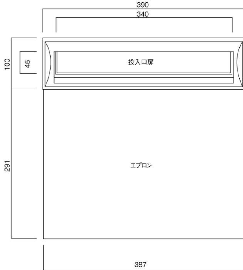
平面図
