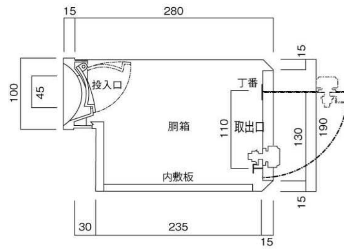
縦断面図
