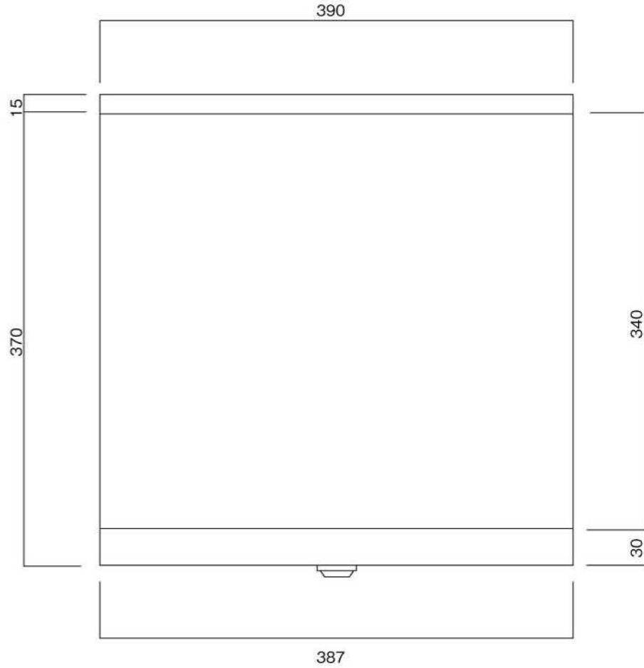
平面図
