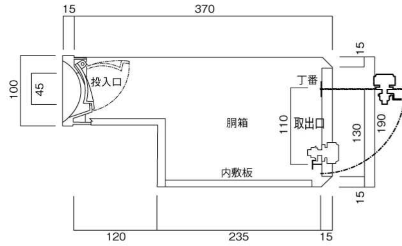
縦断面図
