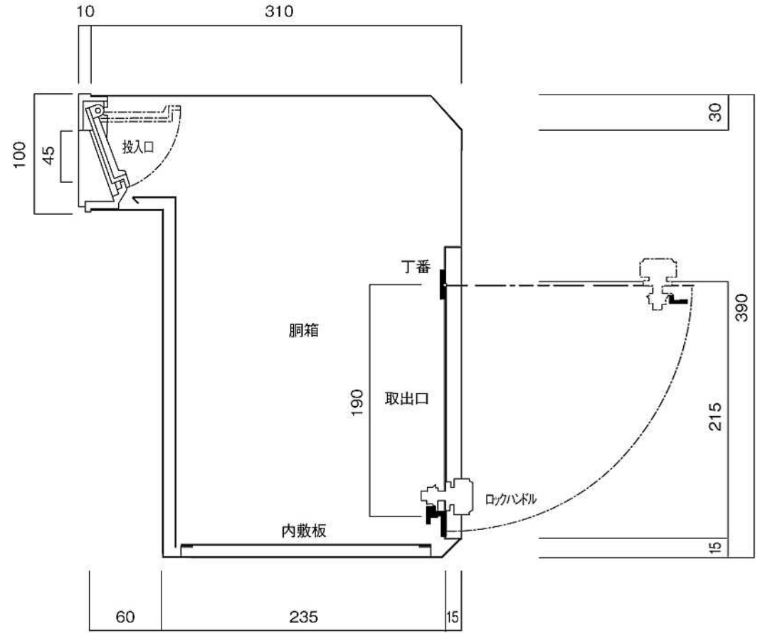
縦断面図
