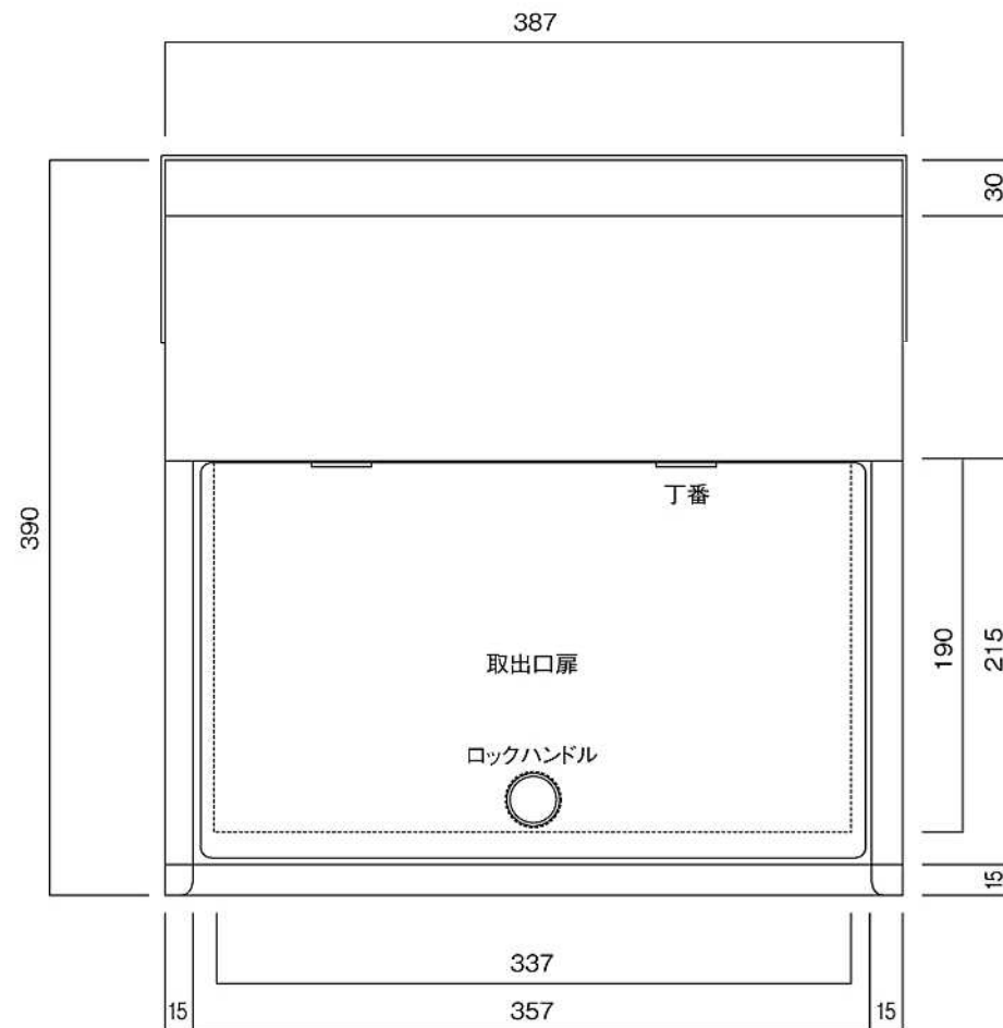
裏面図
