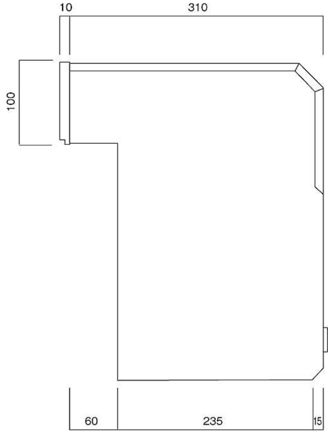
側面図
