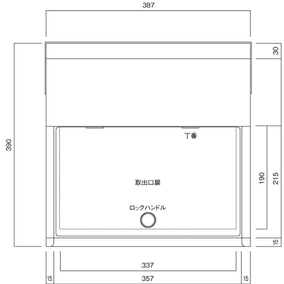
裏面図
