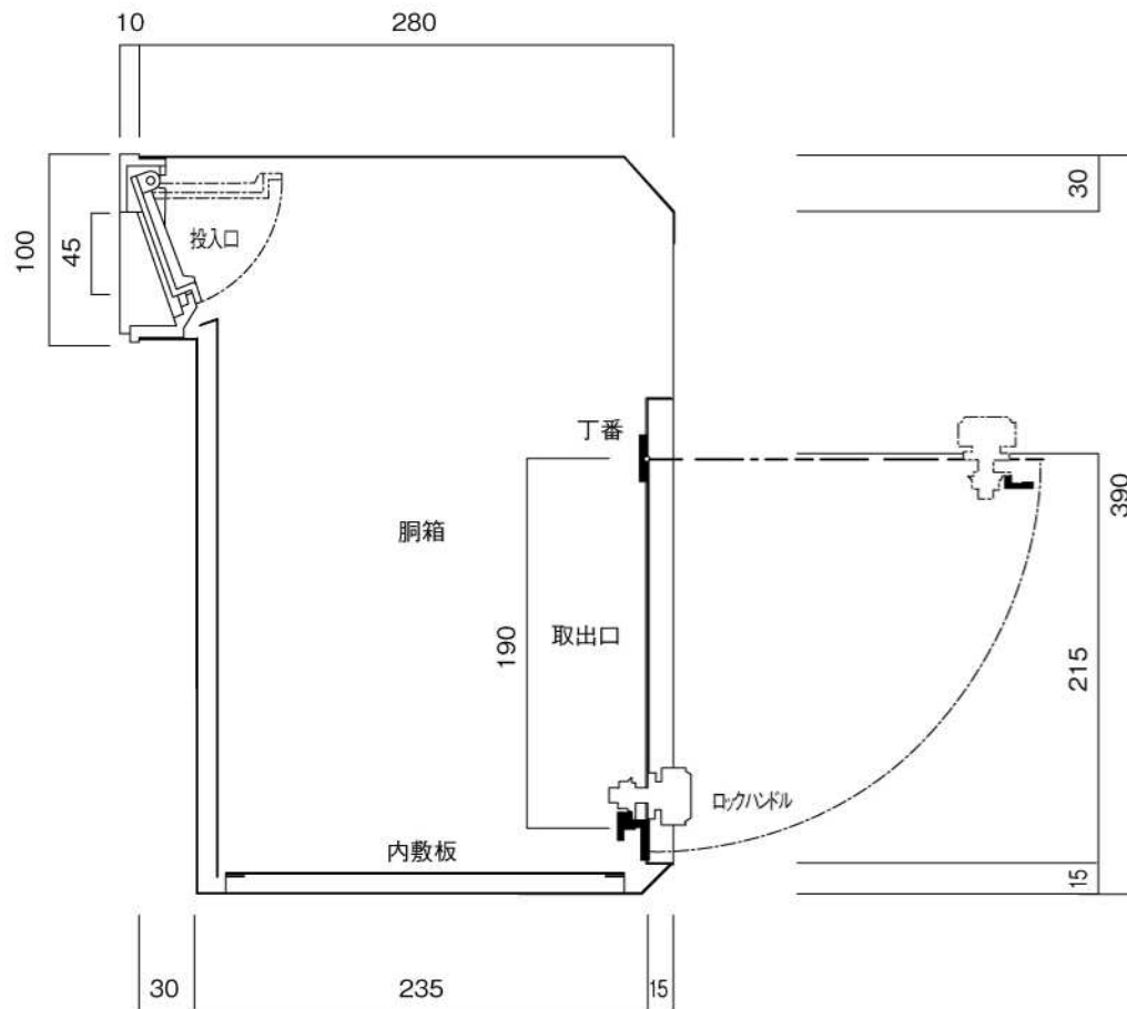
縦断面図
