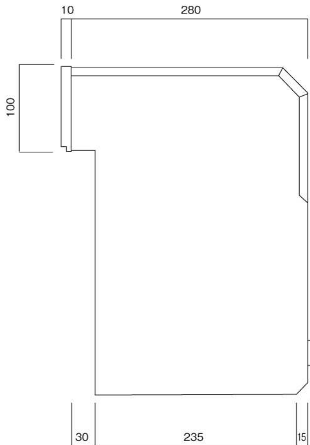
側面図
