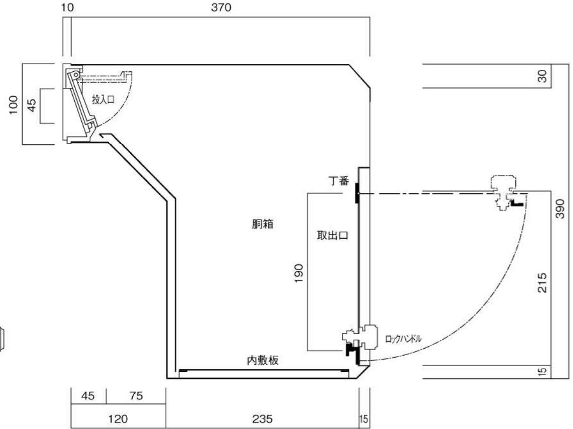
縦断面図
