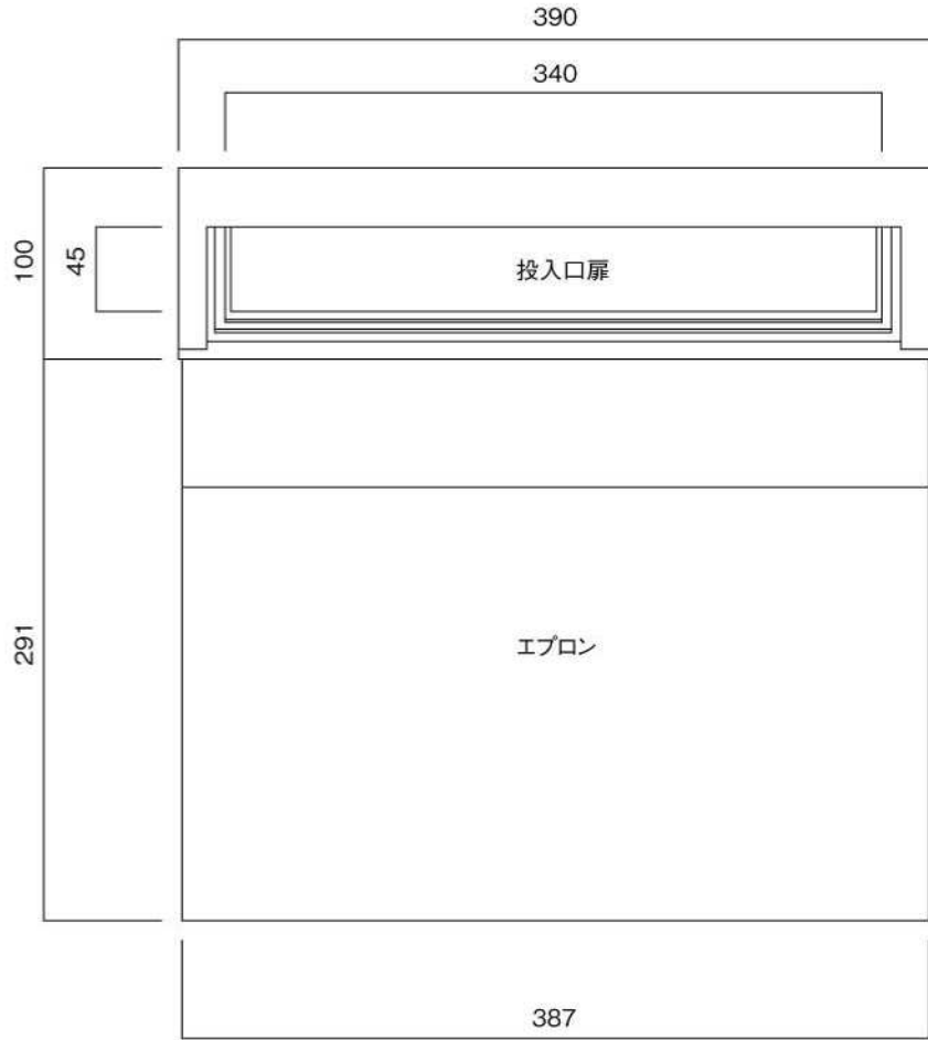
正面図
